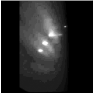
6028 auto | k=502 | phase \Delta=2.0
