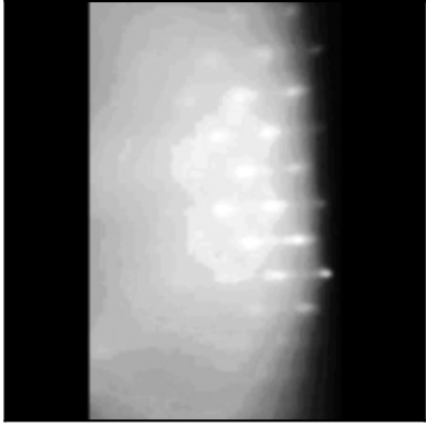
6033 auto | k=363 | phase \Delta=17.2
