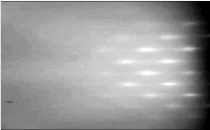
RHEED key-frame ROI
