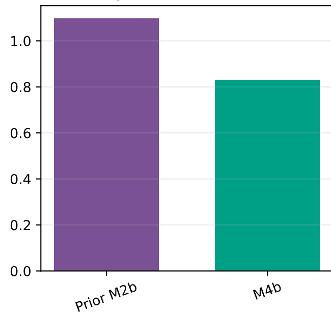
Rq absolute error (nm) ↓
