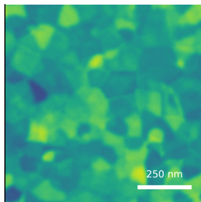
generated AFM Rq=2.47 nm, FSMI=2.02 nm, C=38/100
