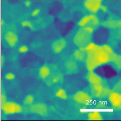
generated AFM Rq=1.53 nm, FSMI=1.26 nm, C=12/100
