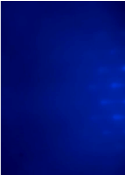
6028 human
