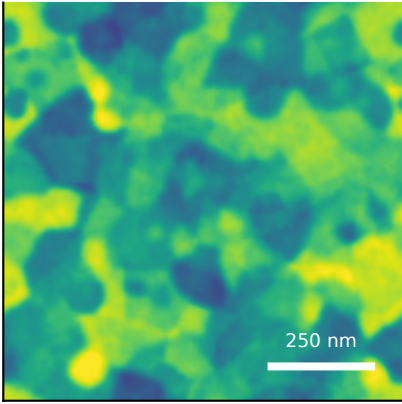
generated AFM Rq=2.55 nm, FSMI=2.21 nm, C=58/100
