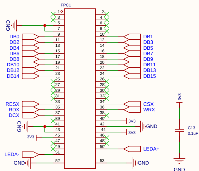
4寸 480*800屏幕 FPC翻盖母座 51P 0.3mm下接
