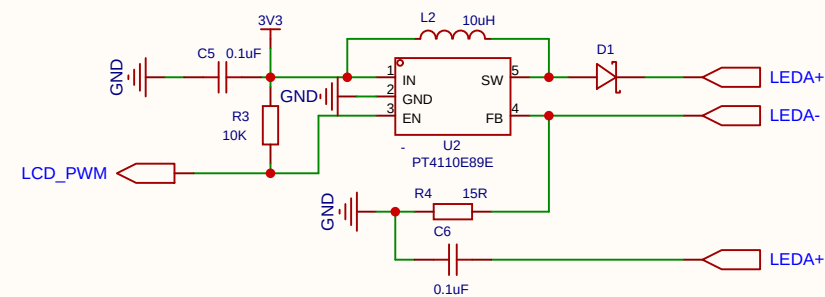
屏幕背光升压
