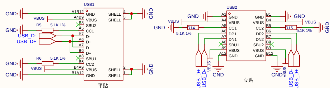
TYPEC接口(根据需要可以二选一或全选)
