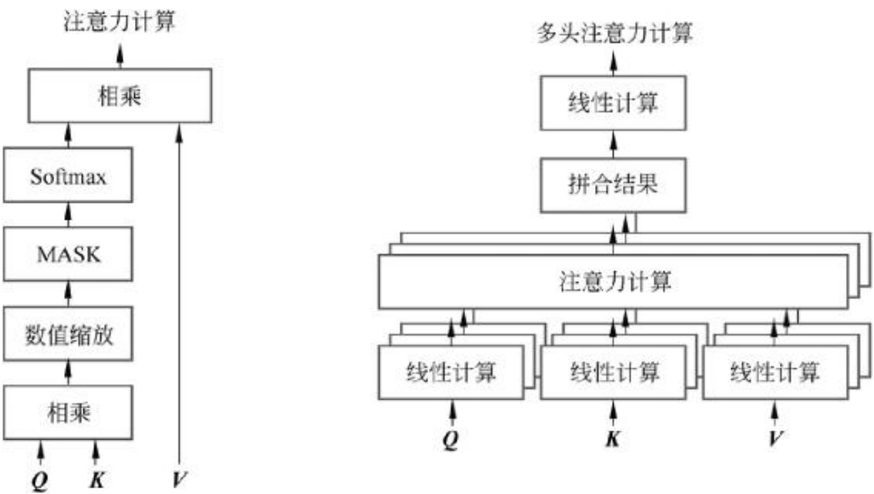
图13-12 单头注意力对比多头注意力
