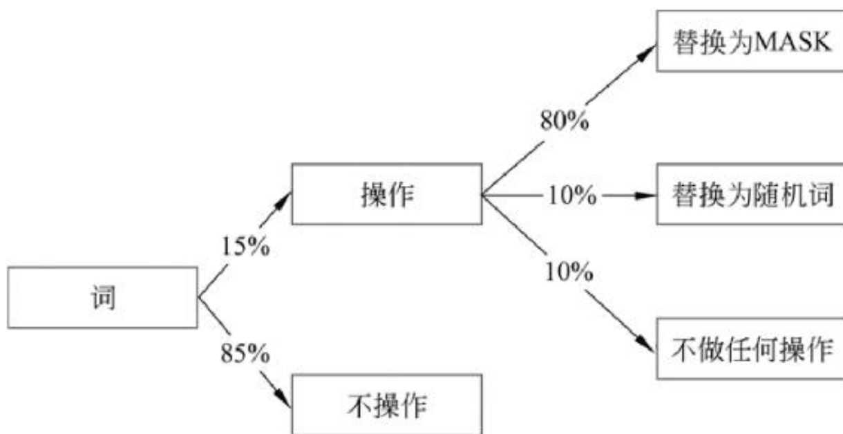
图14-2 random_replace() 函数替换词流程
