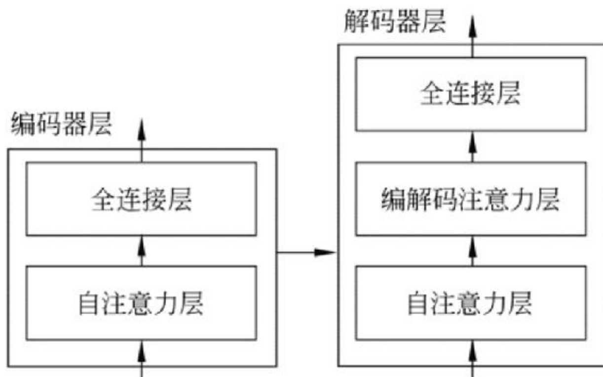
图13-4 编码器和解码器的内部结构
