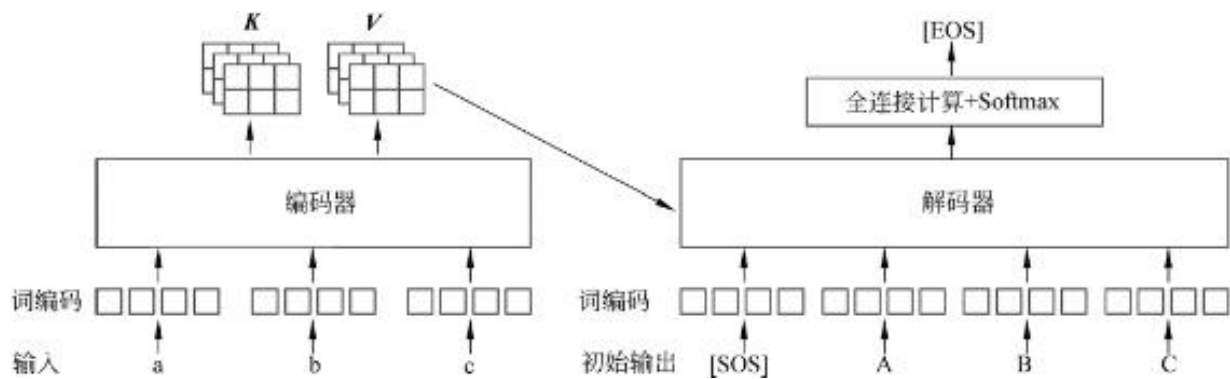
图13-27 解码器解码完成
