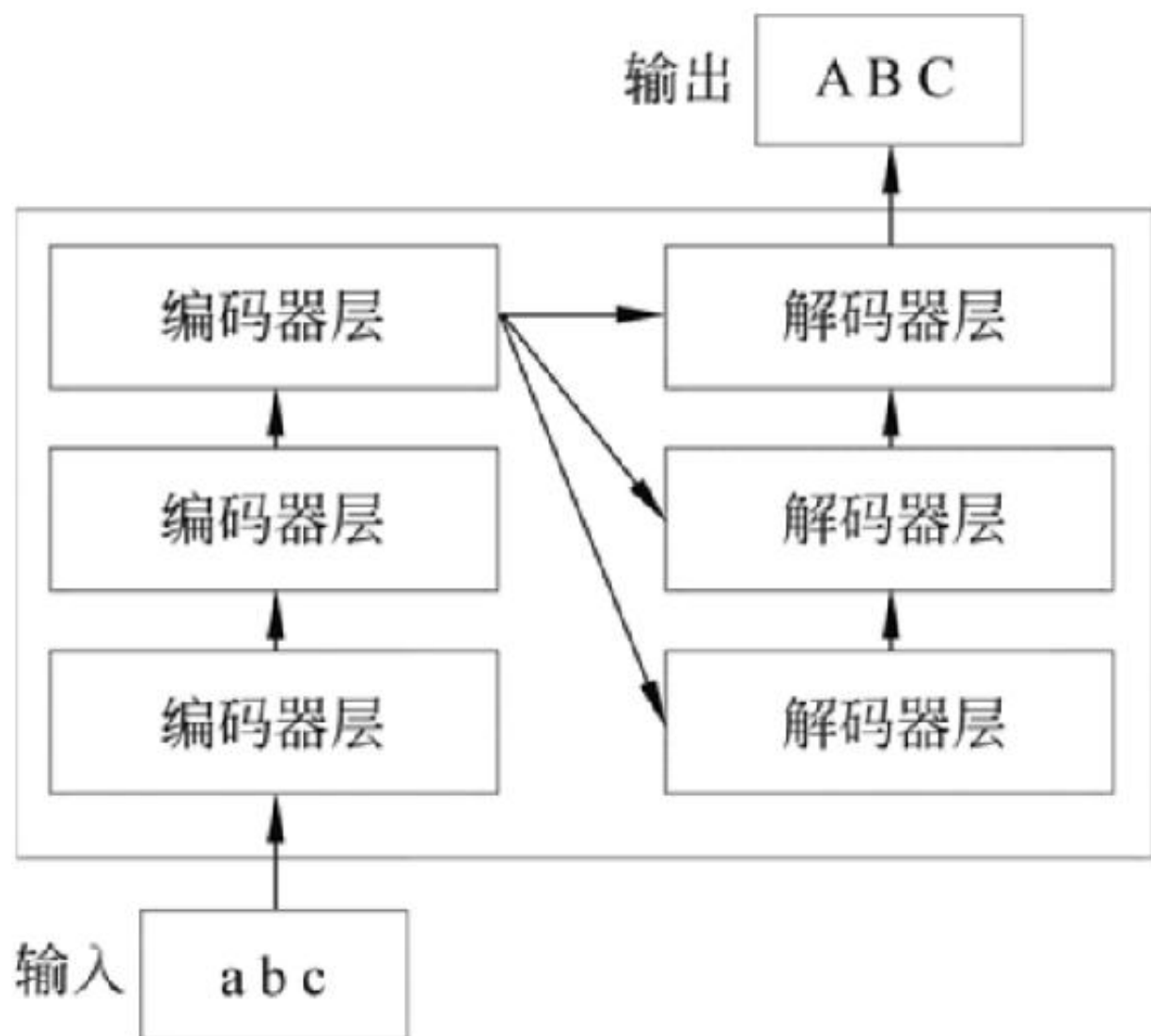
图13-3 编码器和解码器展开图
