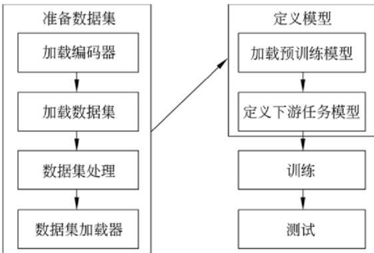
图1-2 针对自然语言处理任务细化的HuggingFace标准研发流程
