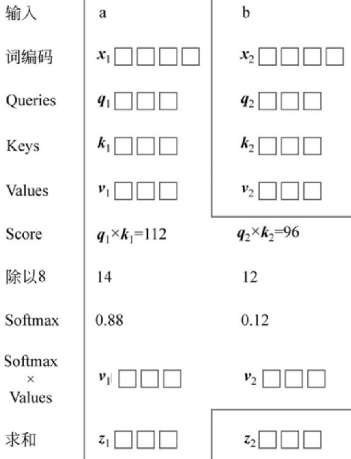
图13-10 自注意力的计算过程
