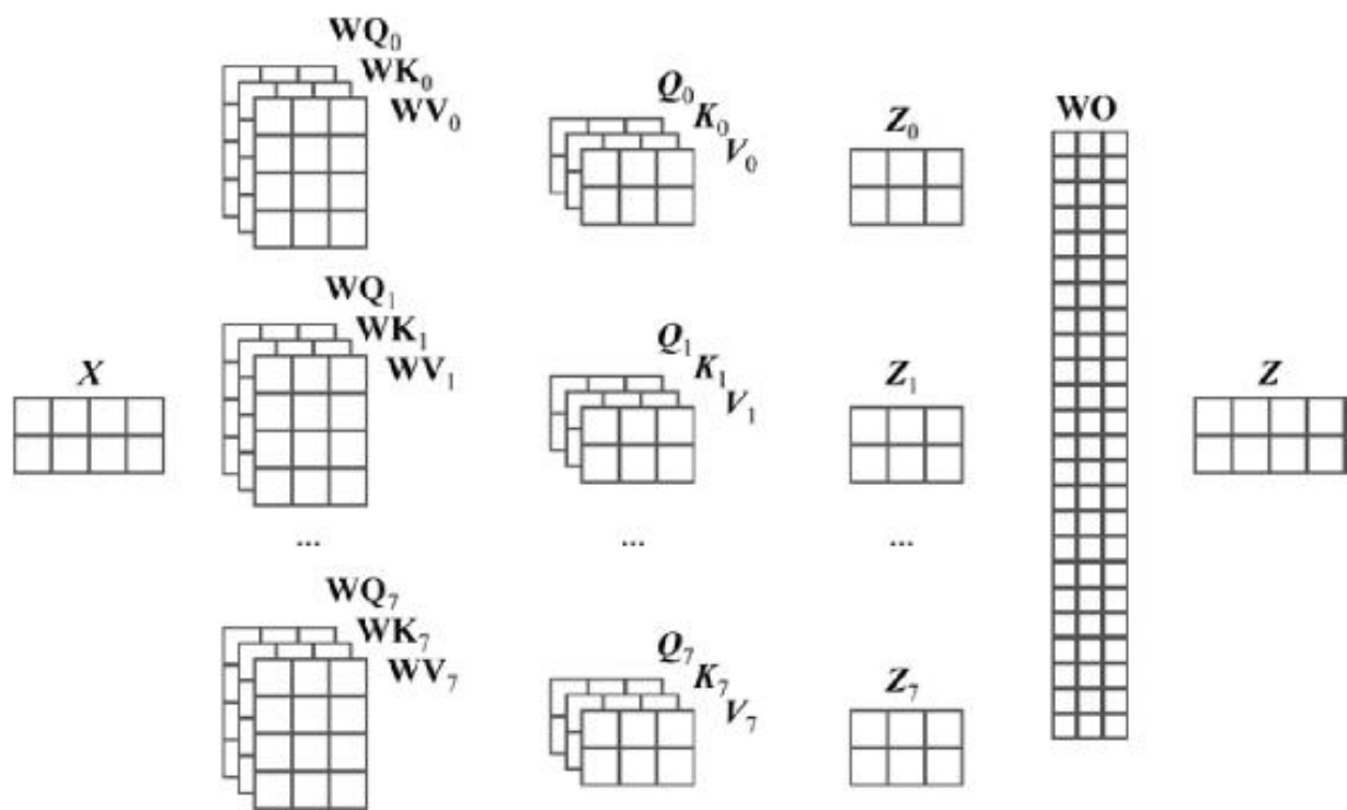
图13-13 多头注意力的完整计算过程
