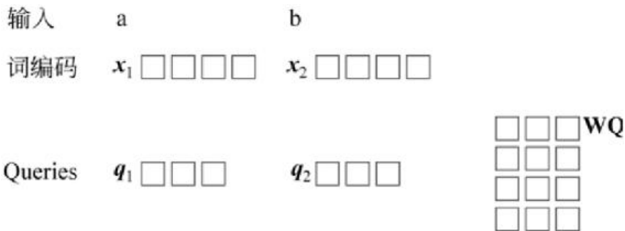
图13-8 使用WQ矩阵投影词向量得到Queries向量
