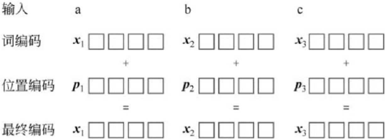
图13-16 在词向量编码中加入位置编码信息
