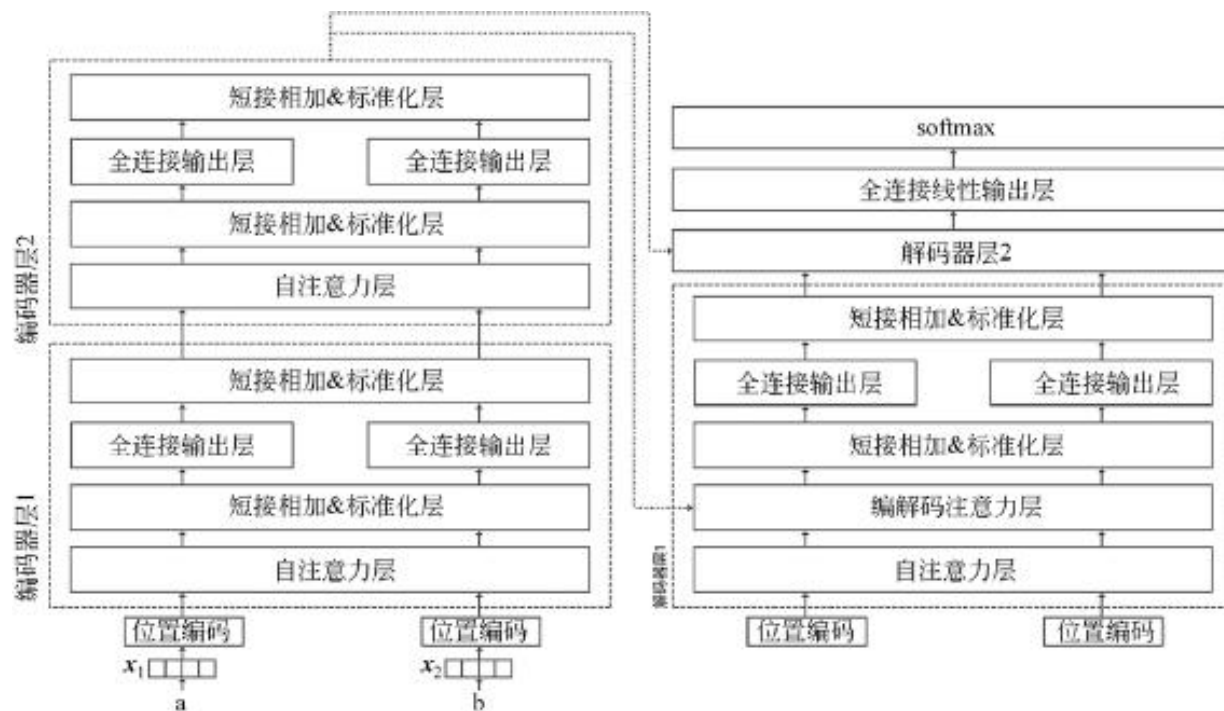
图13-24 Transformer整体计算流程
