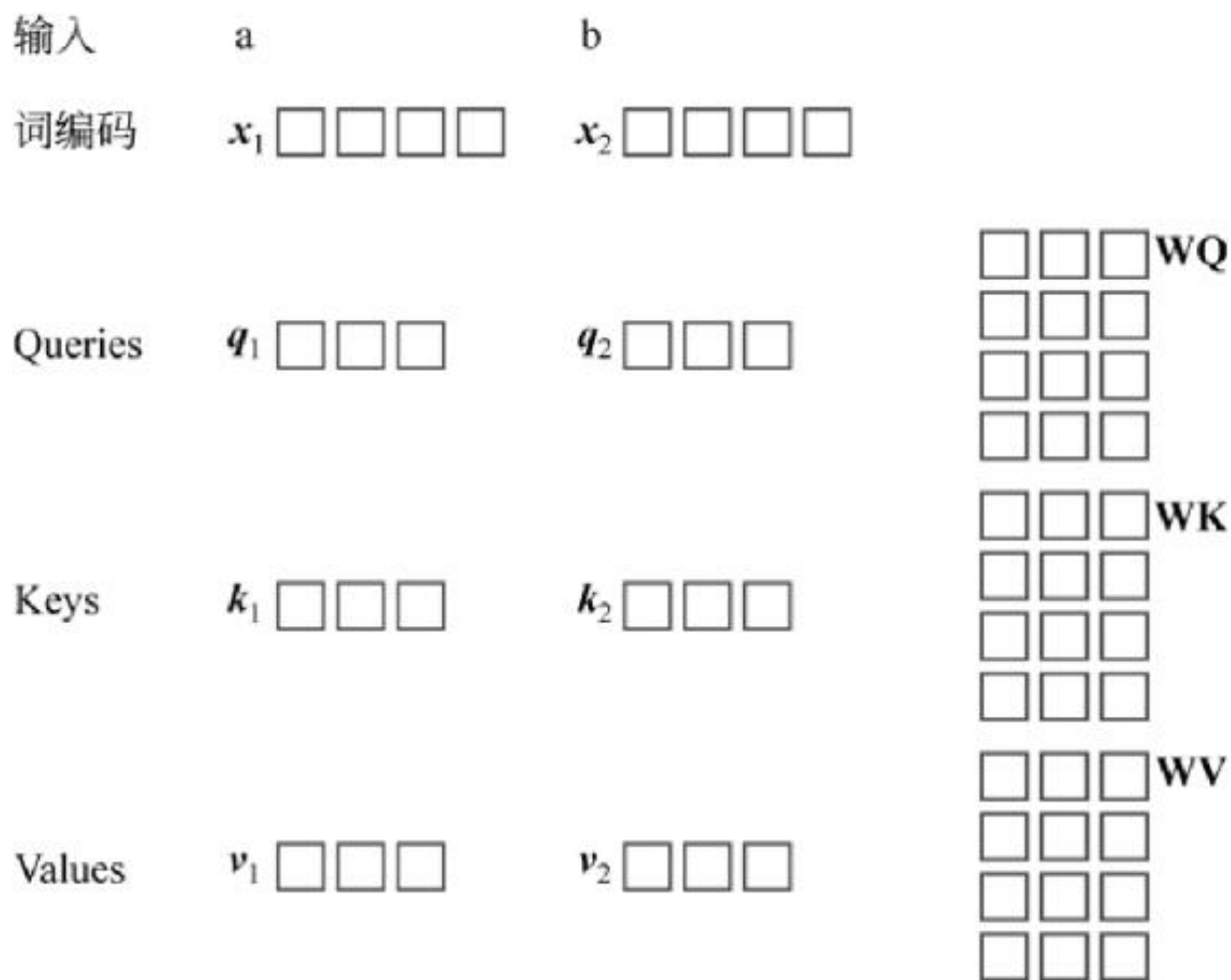
图13-9 生成Queries、Keys和Values词向量
