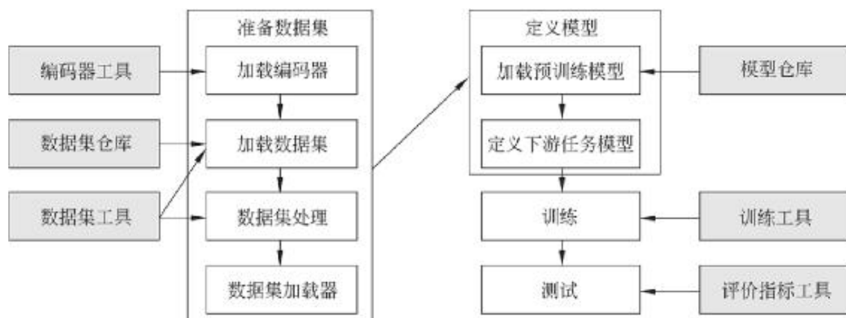
图1-3 各个步骤HuggingFace提供的工具集
