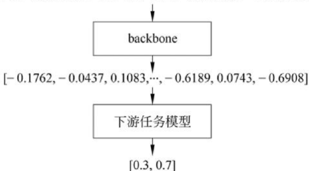
图7-1 使用backbone的网络计算过程
