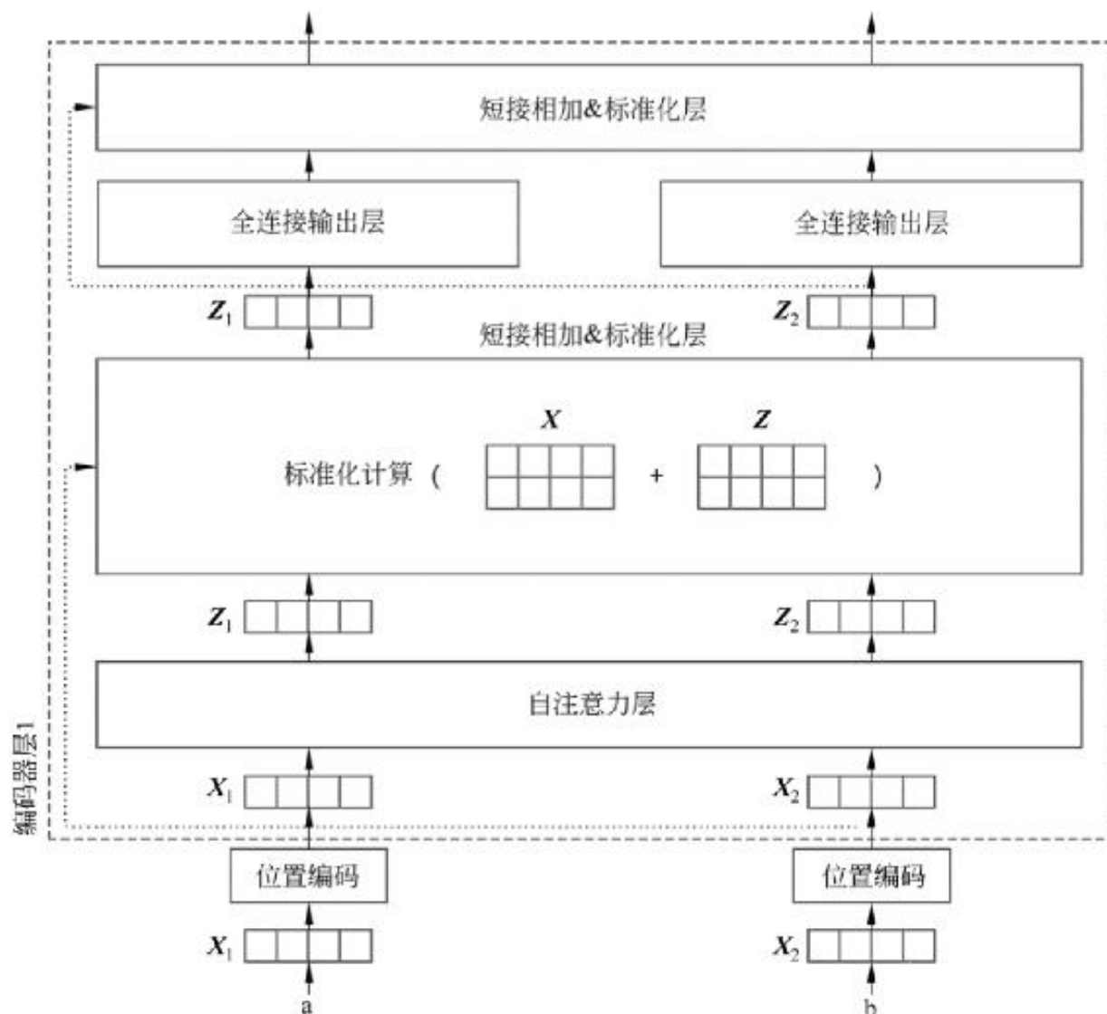
图13-23 编码器计算流程
