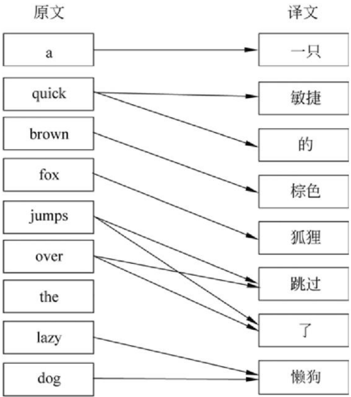
图13-5 自注意力求词与词之间的对应关系
