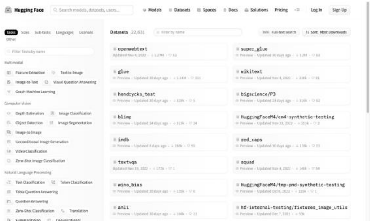
图3-1 HuggingFace数据集页面
