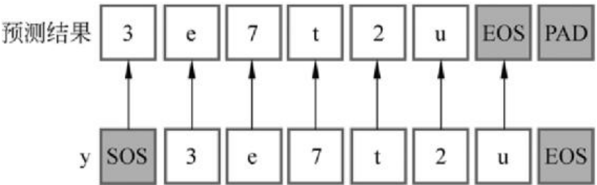
图13-32 y 和预测结果的对应关系
