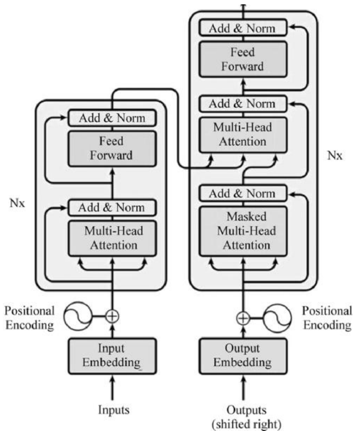
图13-28 Transformer总体架构
