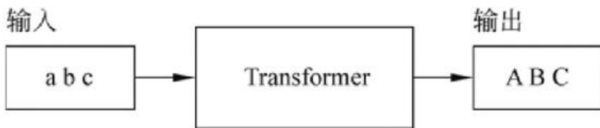
图13-1 黑盒结构
