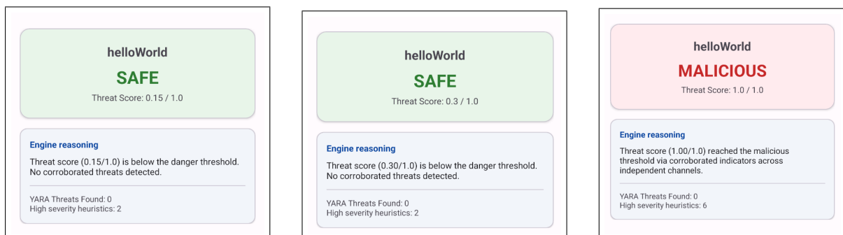
Figura 15: Rapoartele de analiză pentru cele trei versiuni de test cu severitate progresivă
