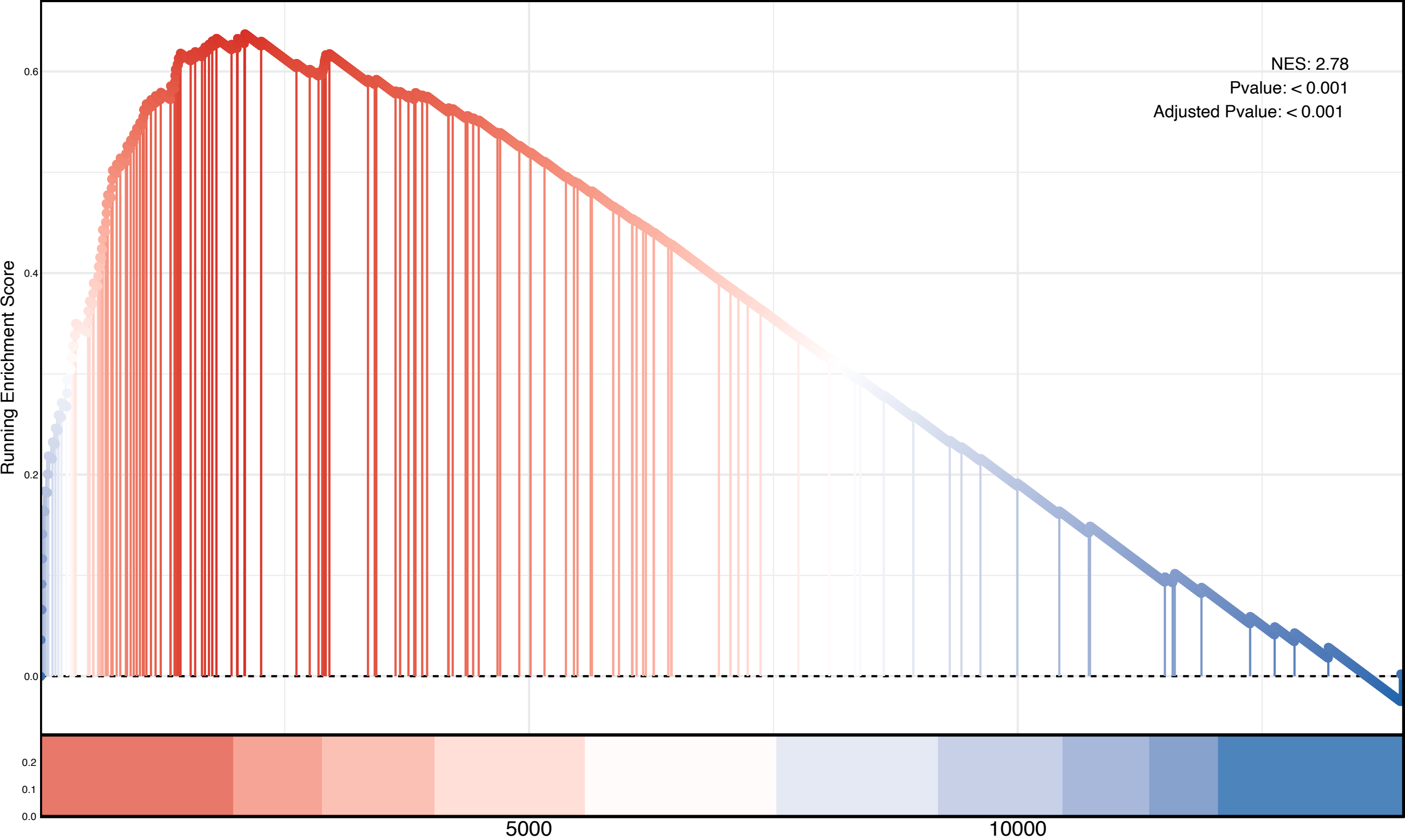
G2 M Checkpoints
