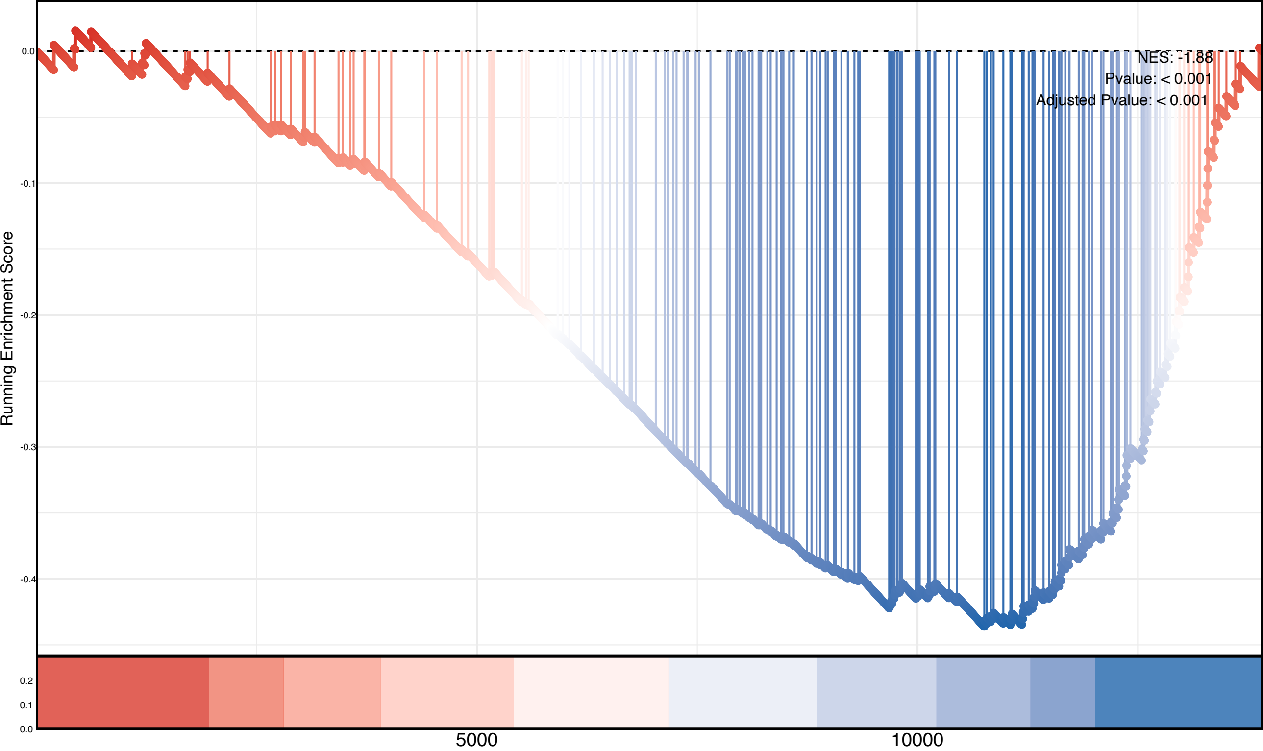
100min Vs 400min IL6 Stim Macrophage Dn
