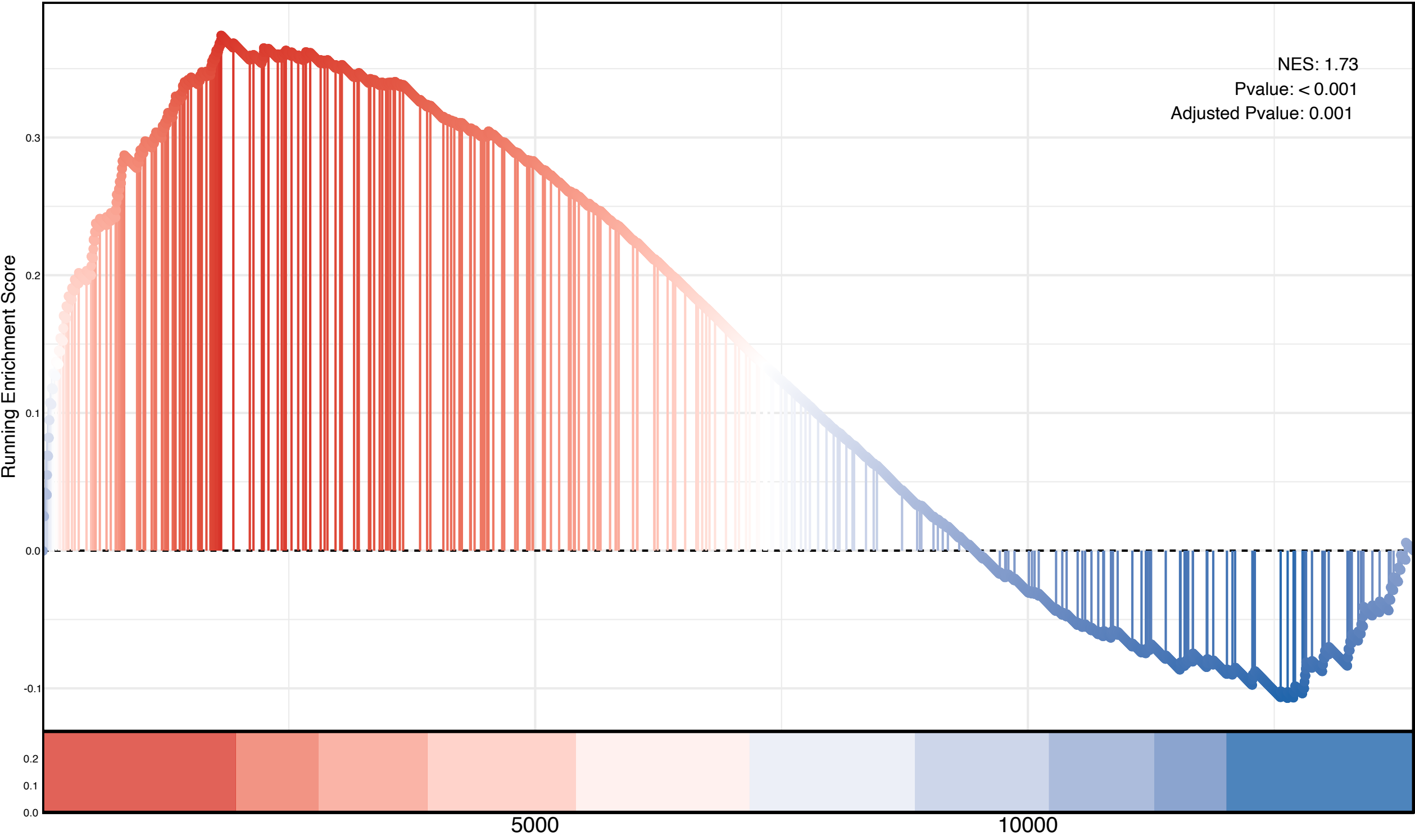
Tef1 Q6
