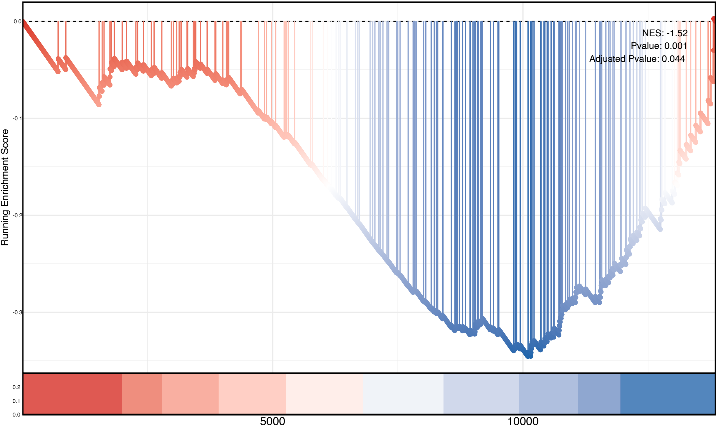
Target Genes
