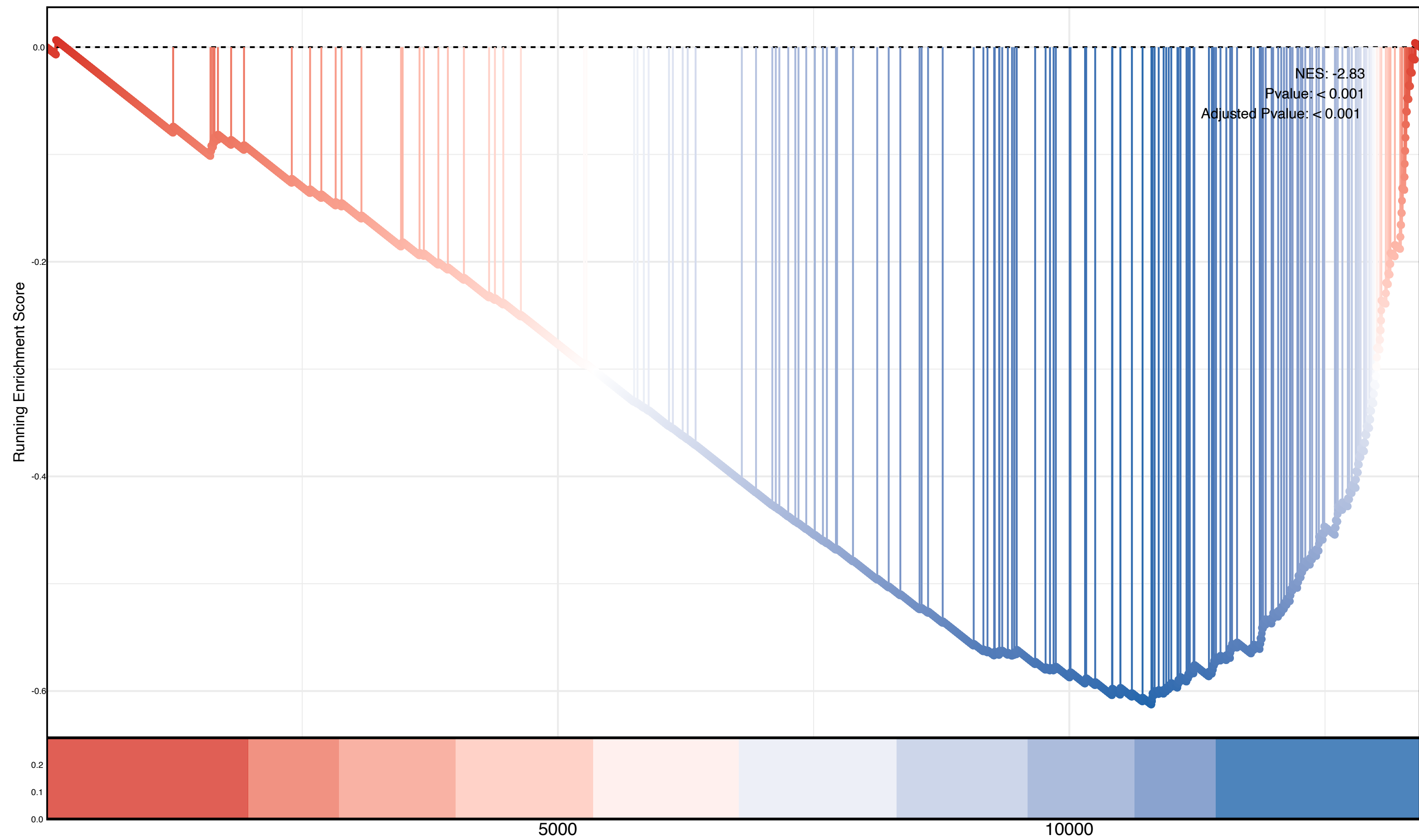
Tconv Vs Treg 24h Tnf Stim Up
