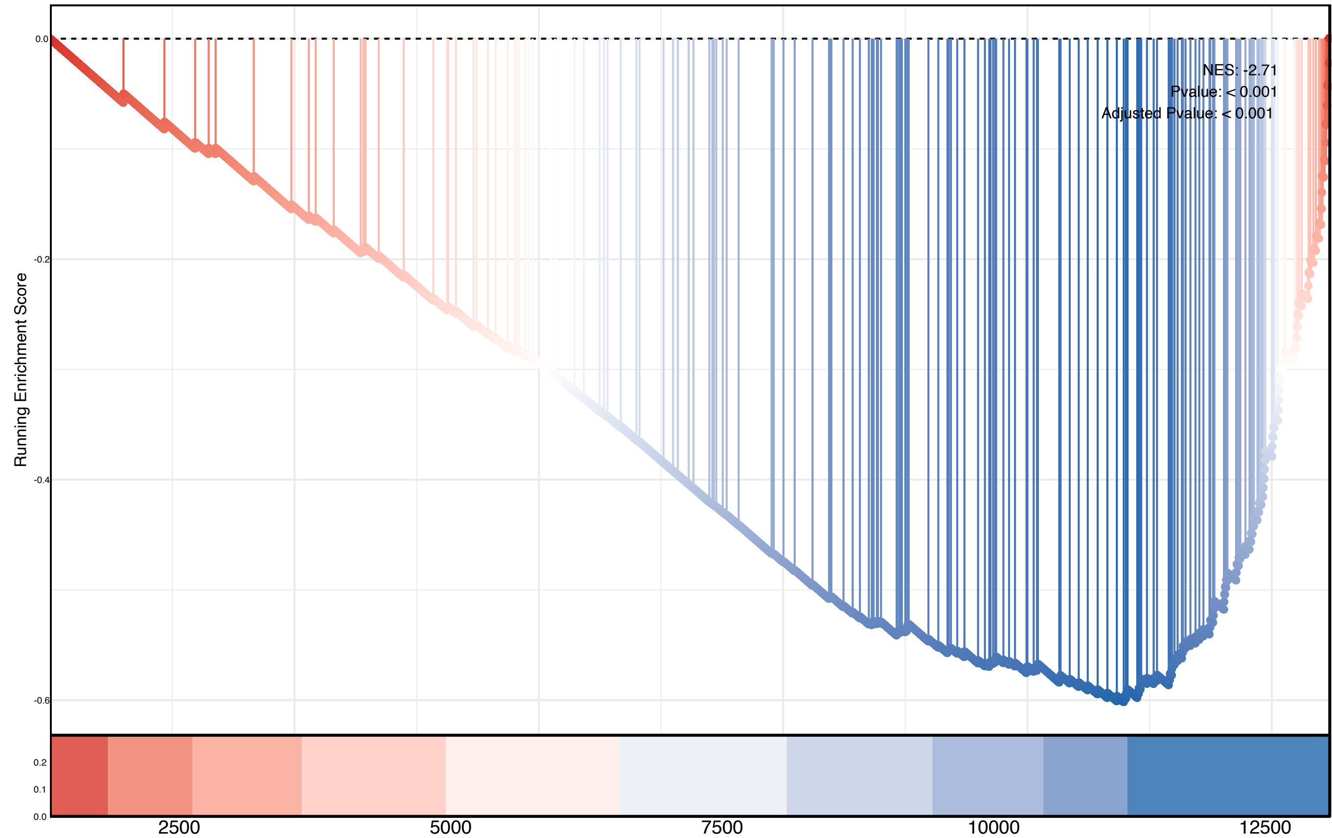
Unstim Vs Il2 Stim Nkcell Dn
