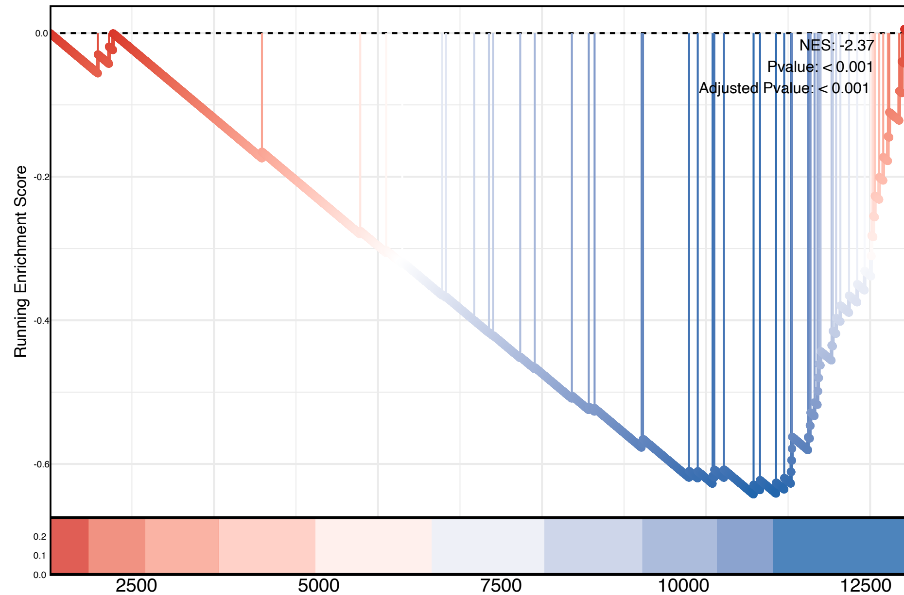
Myc Targets V2
