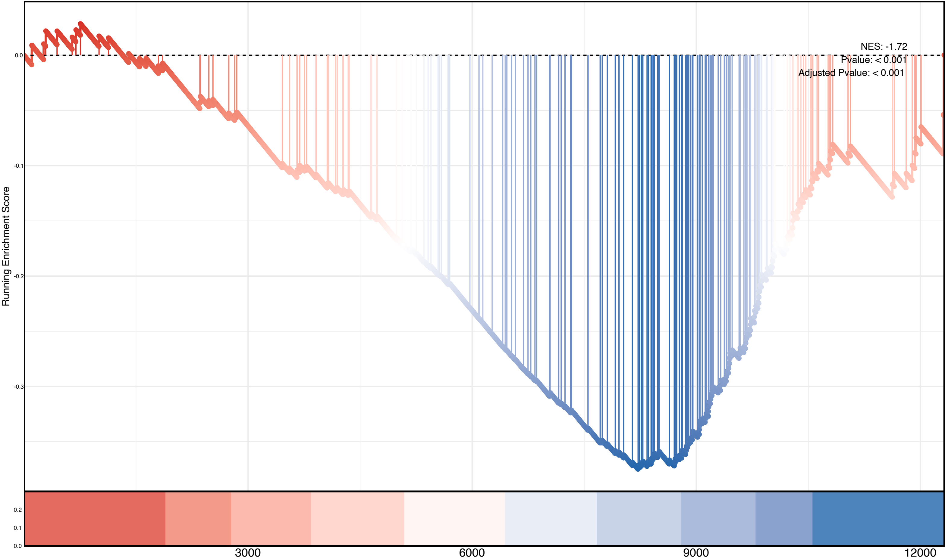
E2f Targets
