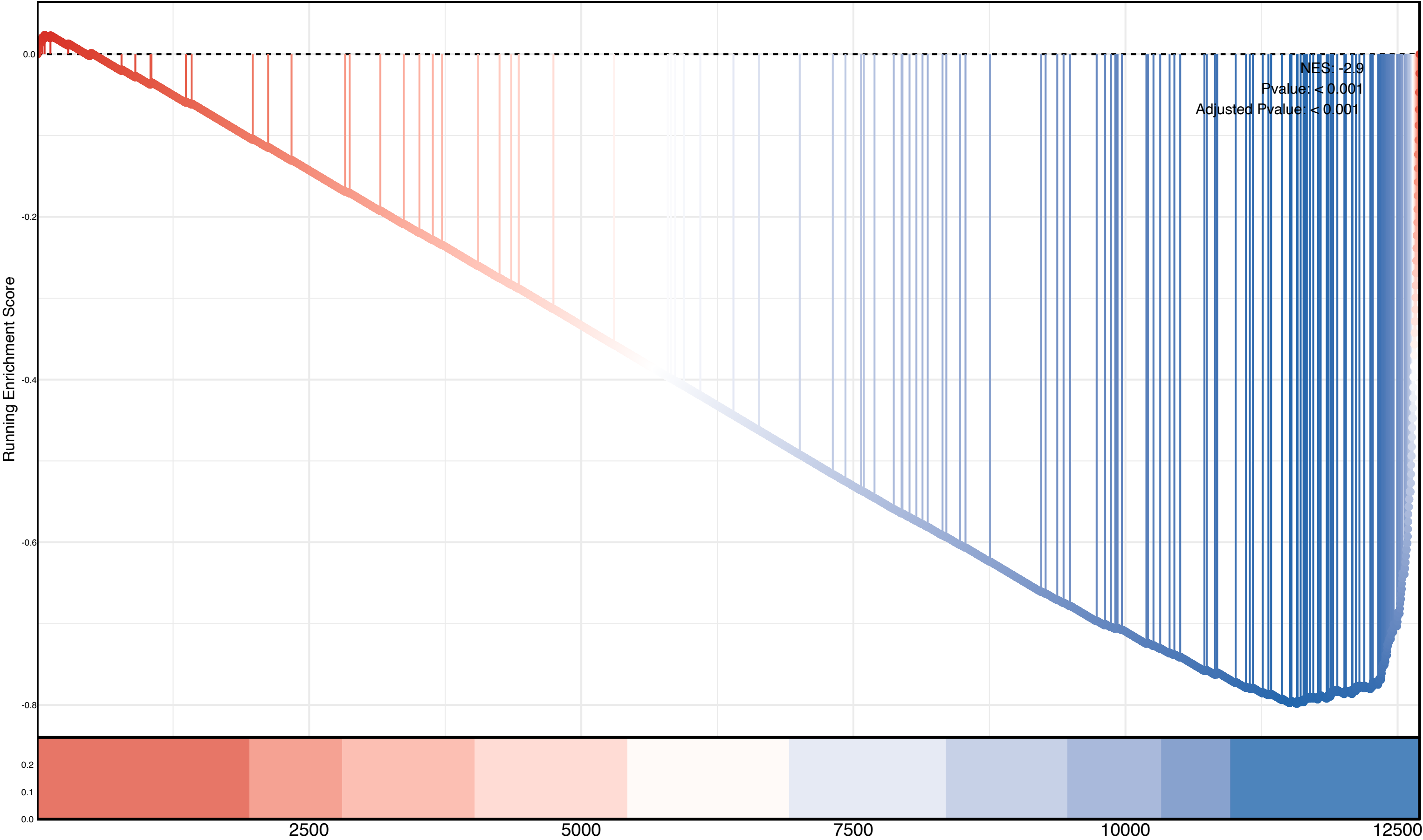
E2f Targets
