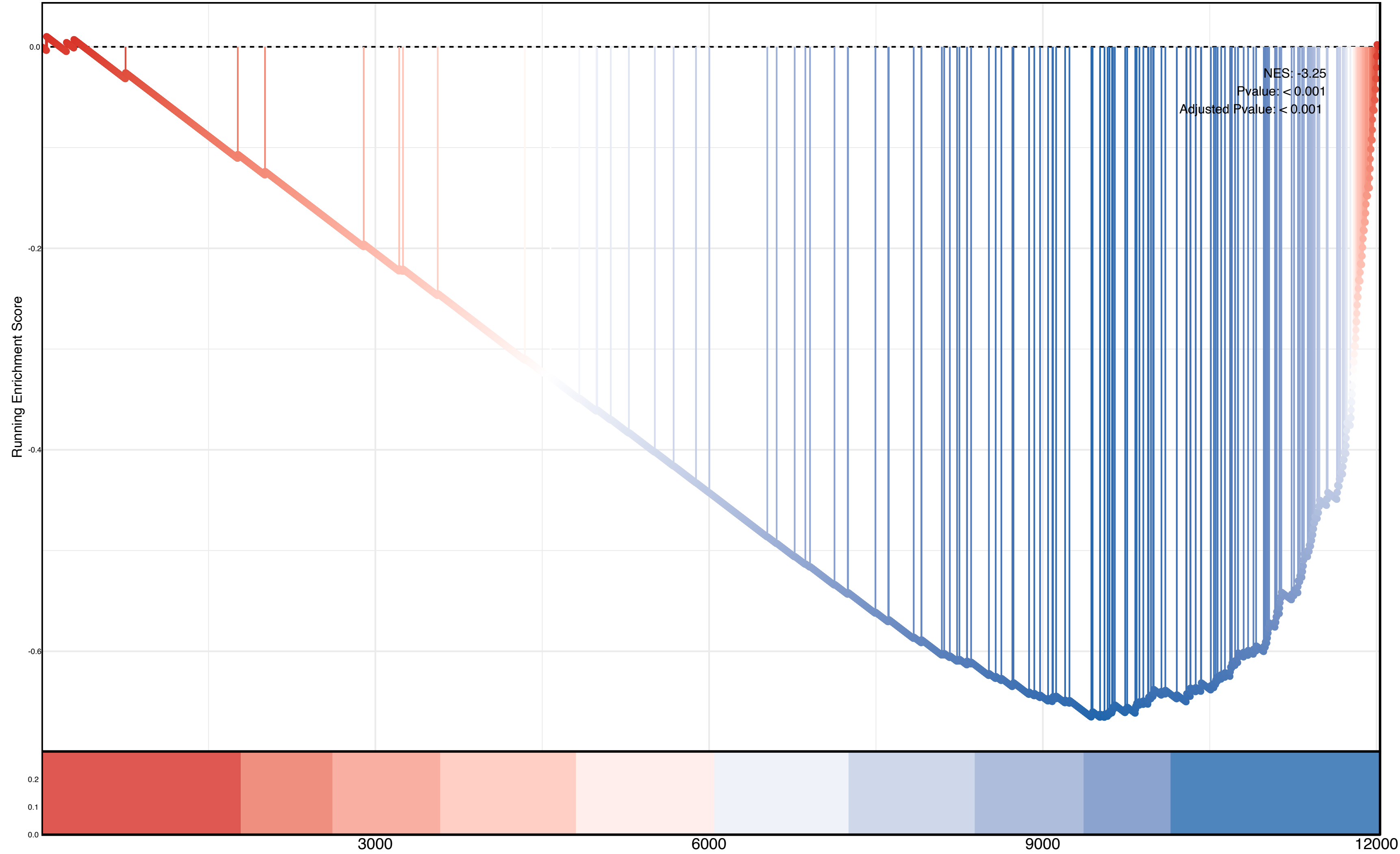
Unstim Vs Il2 Stim Nkcell Dn
