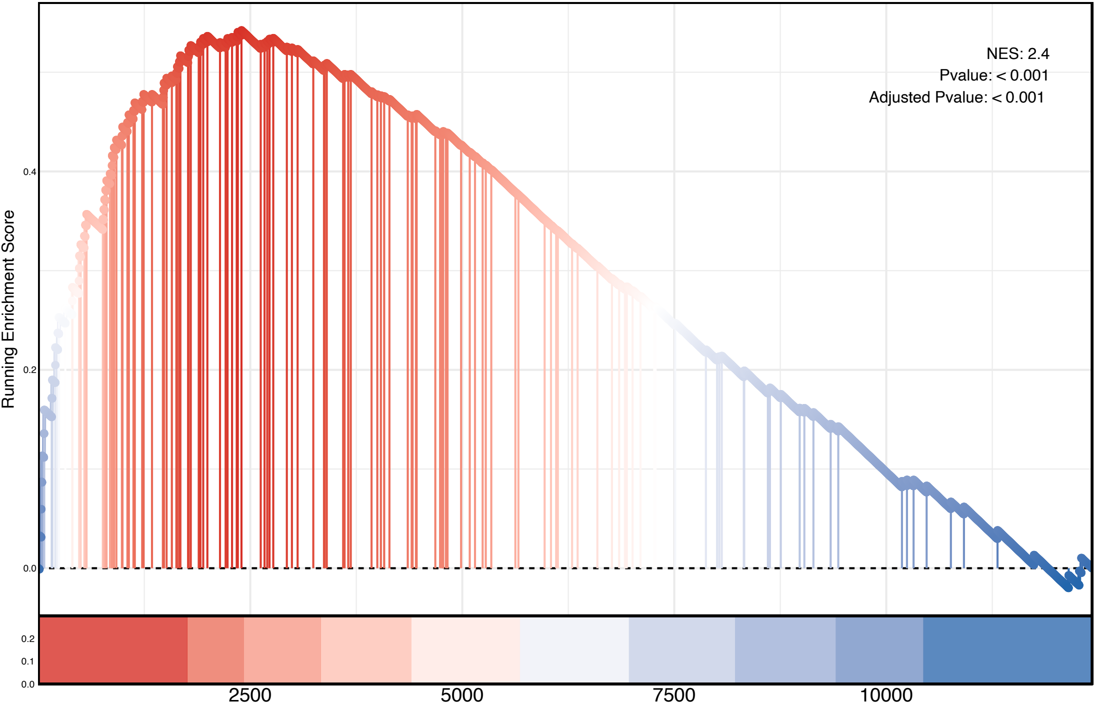
Dn.v1 Up
