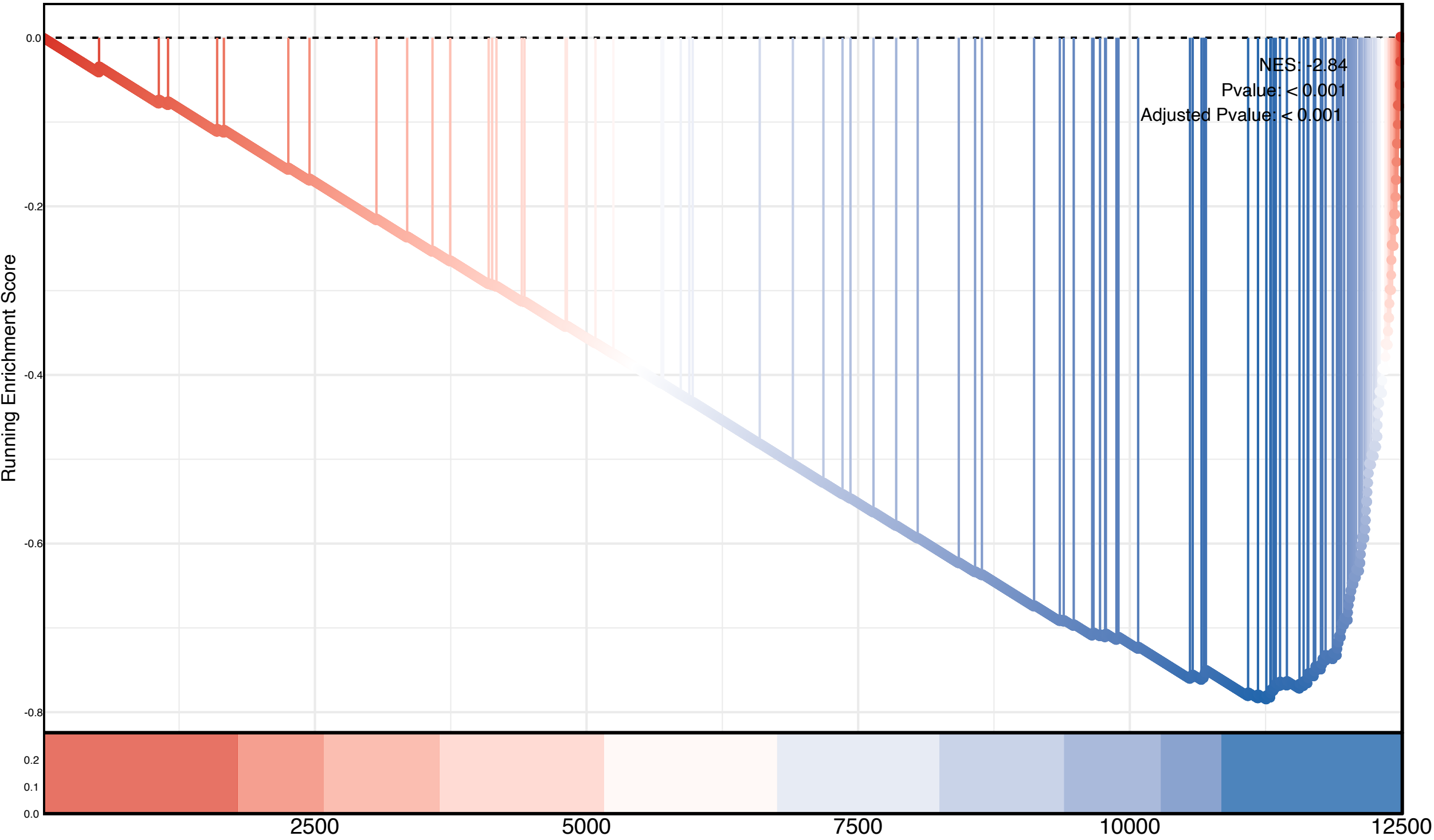
Rho Gtpases Activate Formins
