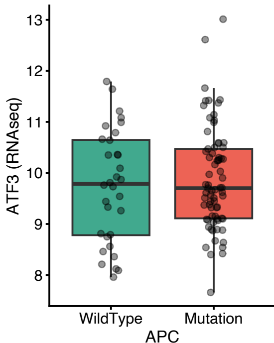
CPTAC-COAD
