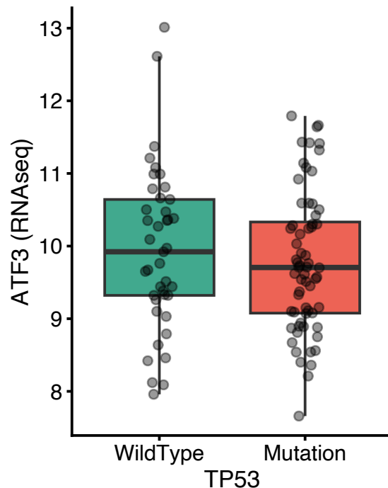
CPTAC-COAD
