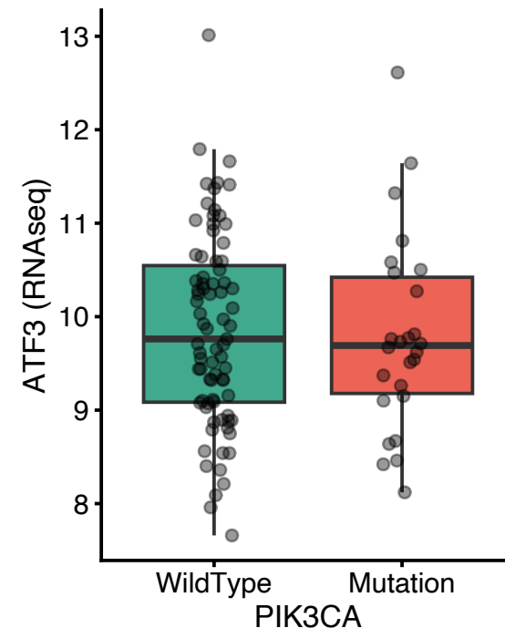
CPTAC-COAD
