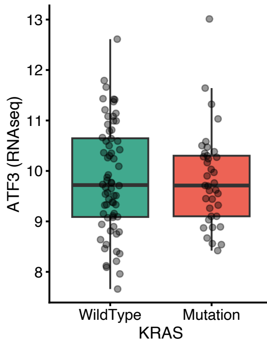
CPTAC-COAD
