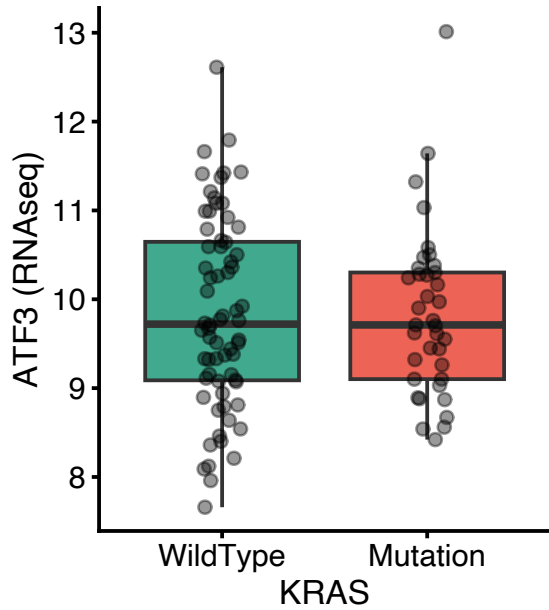
CPTAC-COAD
