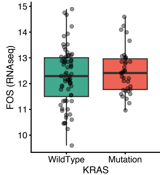
CPTAC-COAD
