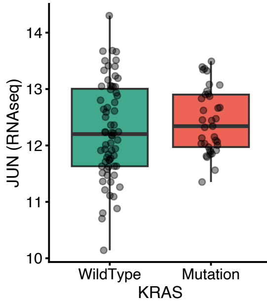
CPTAC-COAD
