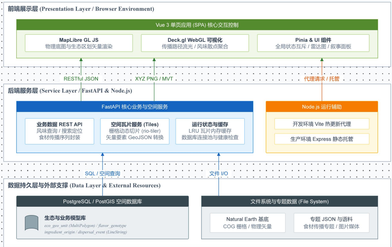
图 3-1 系统总体架构与多层数据交互图 (System Architecture & Data Flow)
