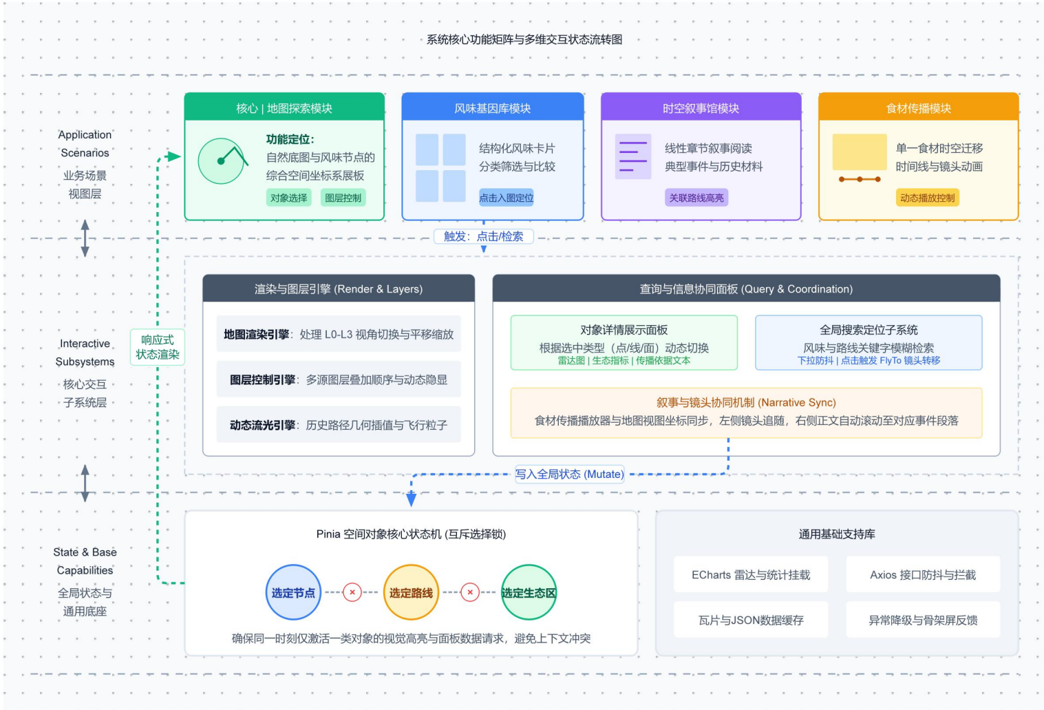
图 8 系统模块划分与各模块多维状态交互示意图
