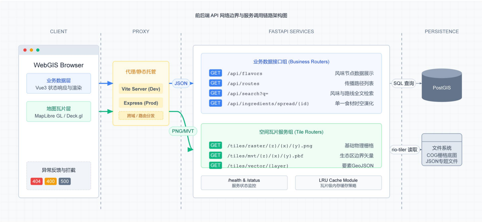
图 9 系统结构设计：前后端 API 网络边界与服务调用链路架构图
