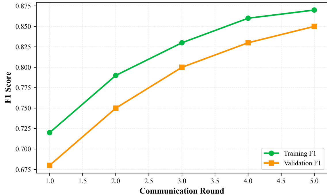
(b) F1 Score Progression
