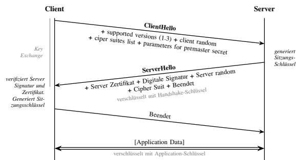
Abbildung 1. TLS 1.3 Handshake
