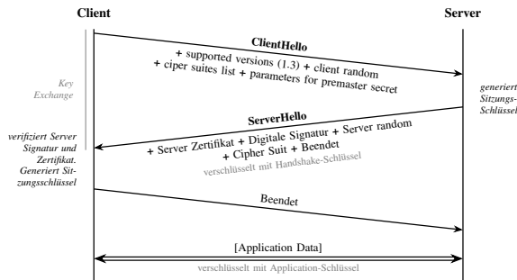
Abbildung 1. TLS 1.3 Handshake
