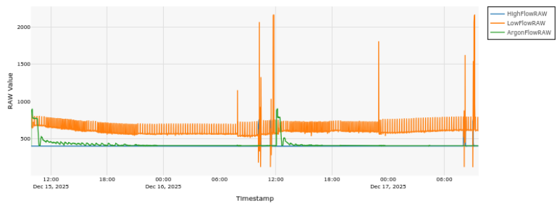
RAW Gas Sensor Values
