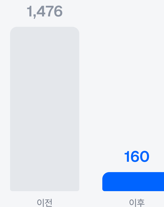
AI에 넘긴 도구 설명 분량 (토큰)
