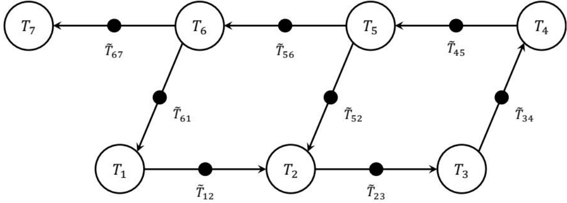
图 6.1: 图 6.2 位姿图示例。这里，顶点与待估未知位姿 T_i = (t_i, R_i) \in \text{SE}(d) 一一对应；有向边则与它们之间相对位姿的一组带噪测量 \tilde{T}_{ij} \approx T_i^{-1} T_j 一一对应。
