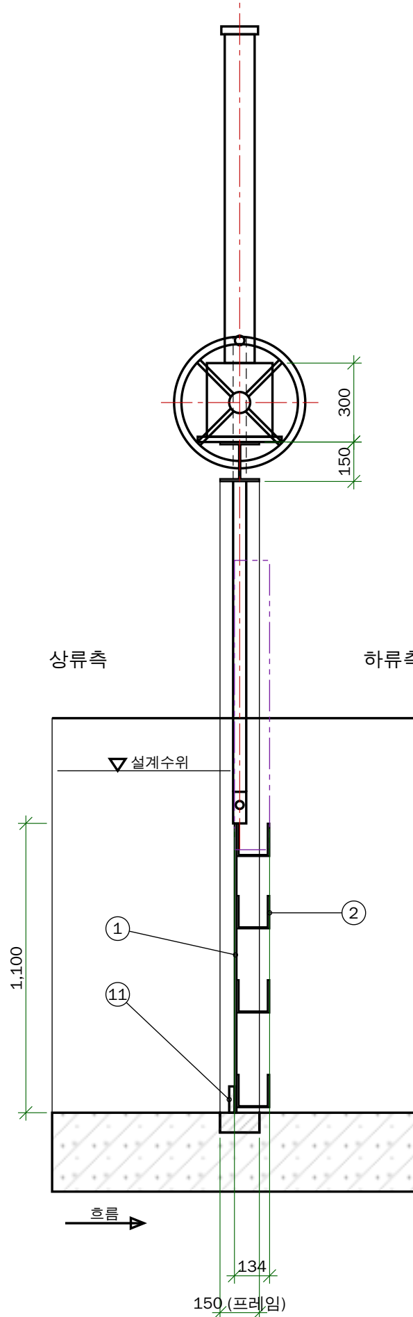
단면도 A-A S=1:20
