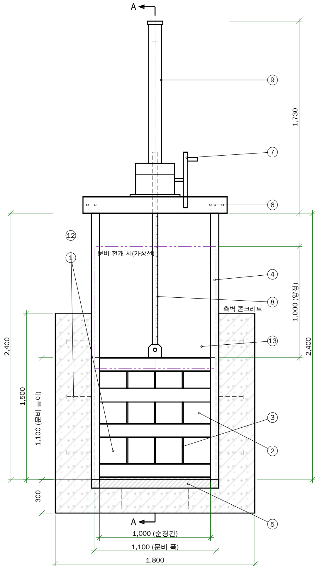
정면도 (하류측에서 봄) S=1:20
