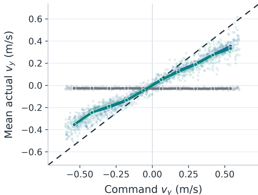
(e) v_y tracking error
