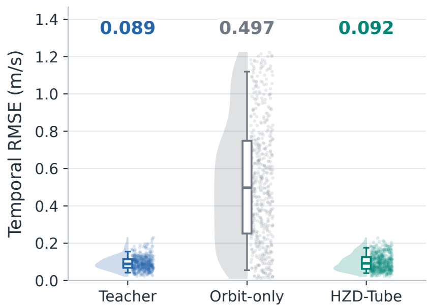
(d) v_x tracking error
