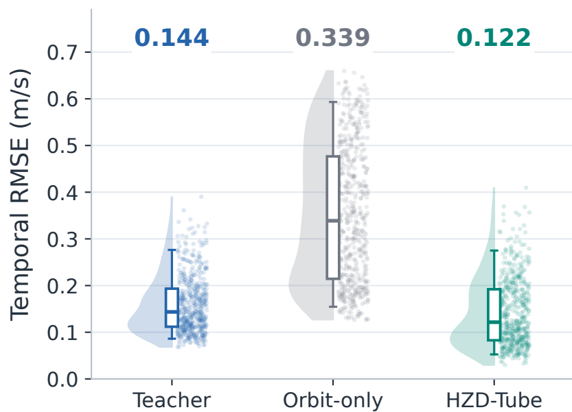
(e) v_y tracking error
