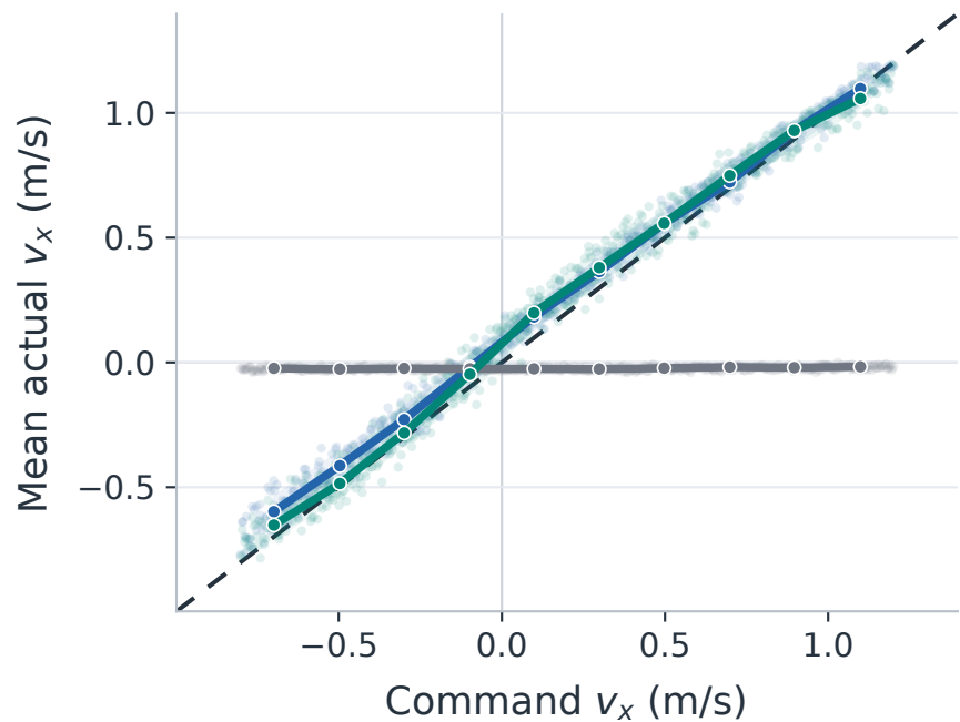
(d) v_x tracking error
