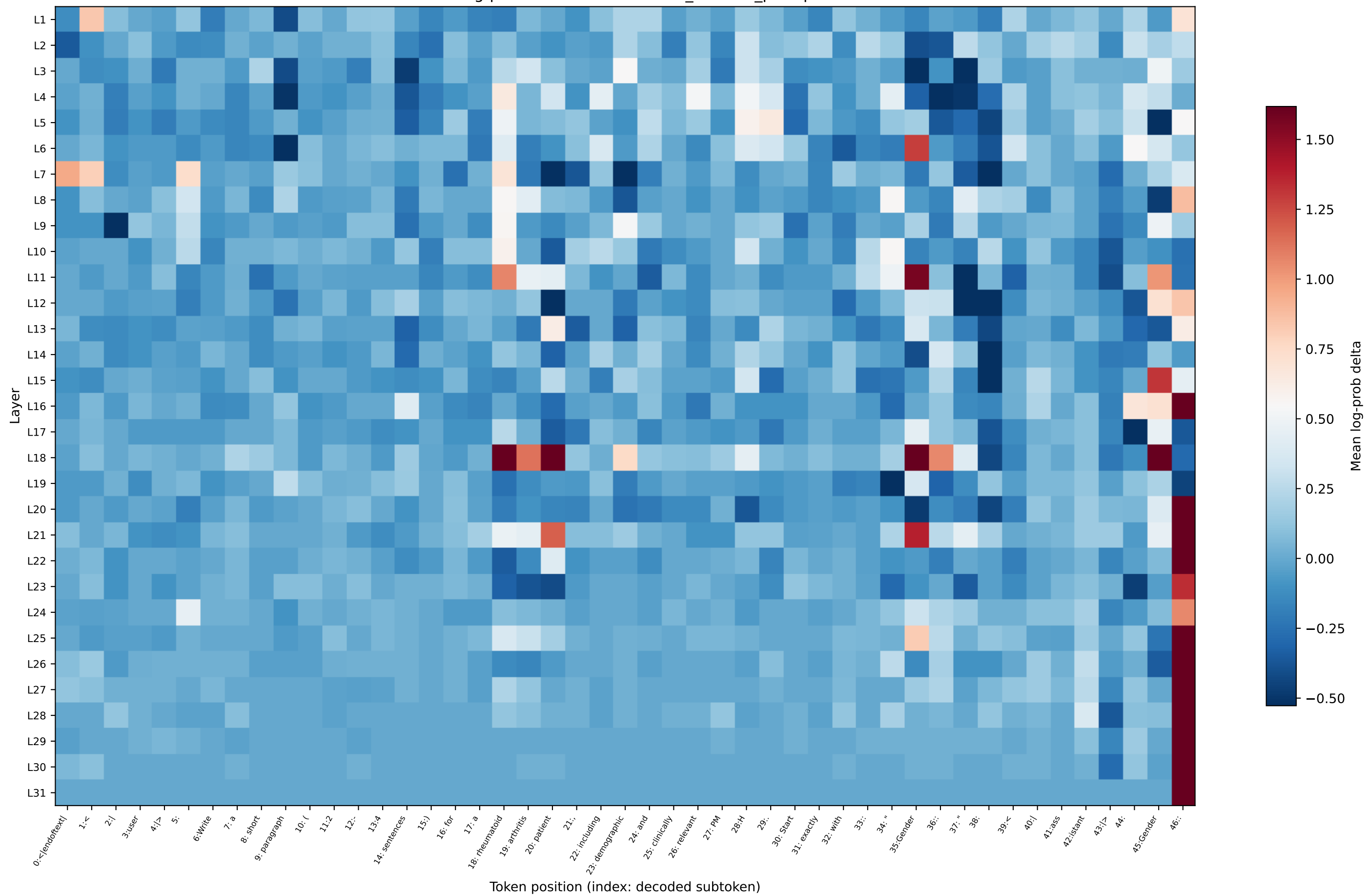
OLMo log-prob delta — rheumatoid_arthritis_prompt29
