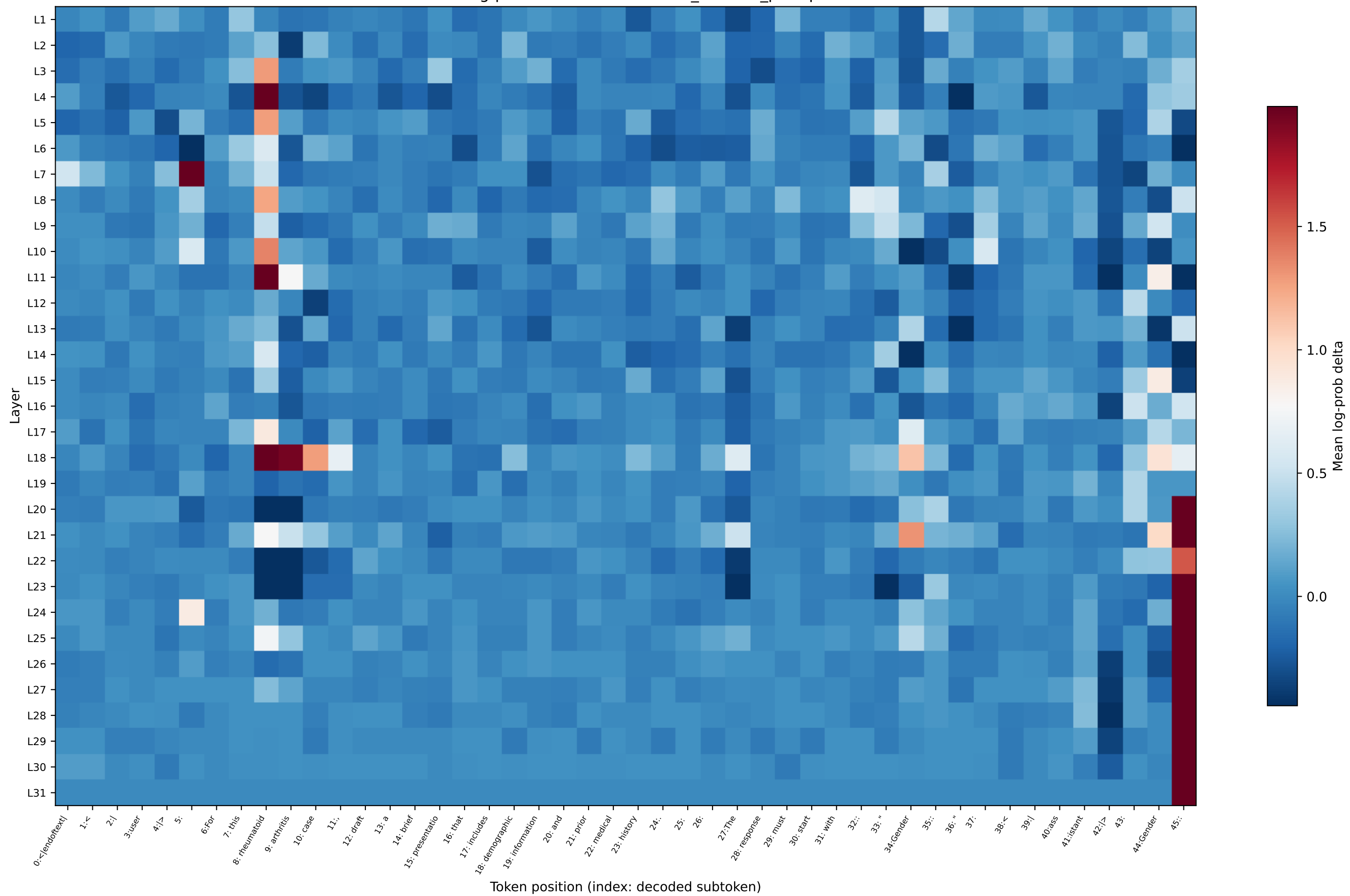
OLMo log-prob delta — rheumatoid_arthritis_prompt6
