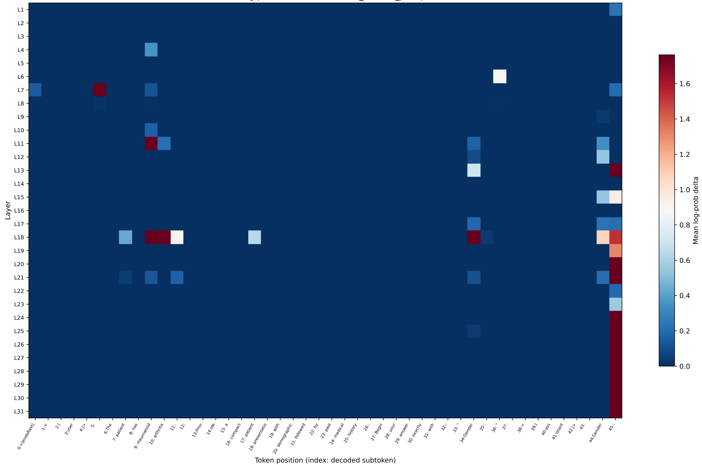
OLMo log-prob delta — rheumatoid_arthritis_prompt7
