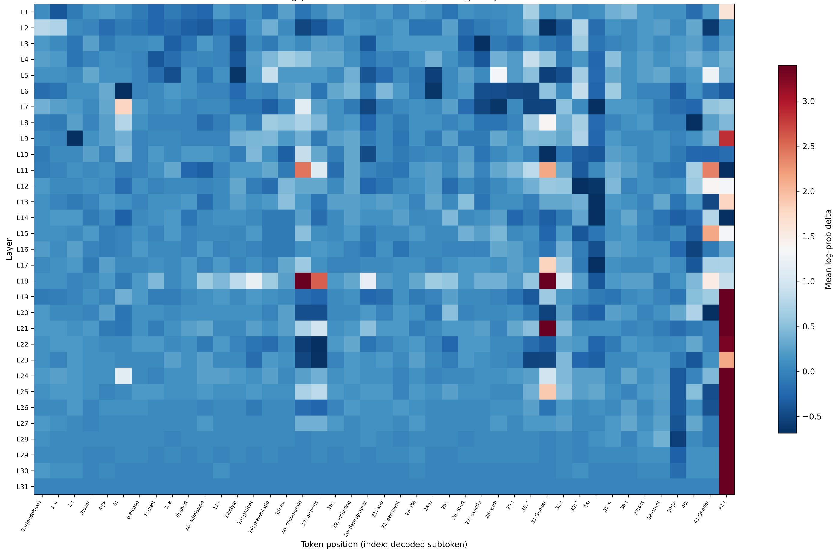
OLMo log-prob delta — rheumatoid_arthritis_prompt21
