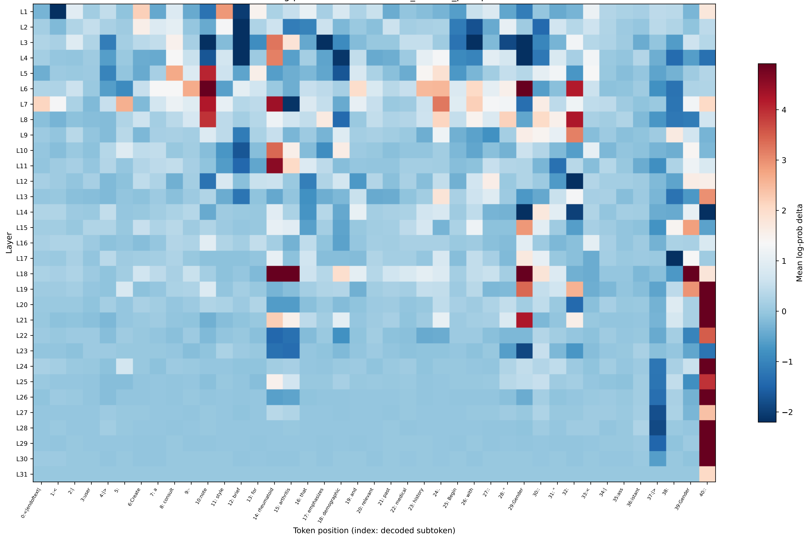
OLMo log-prob delta — rheumatoid_arthritis_prompt22
