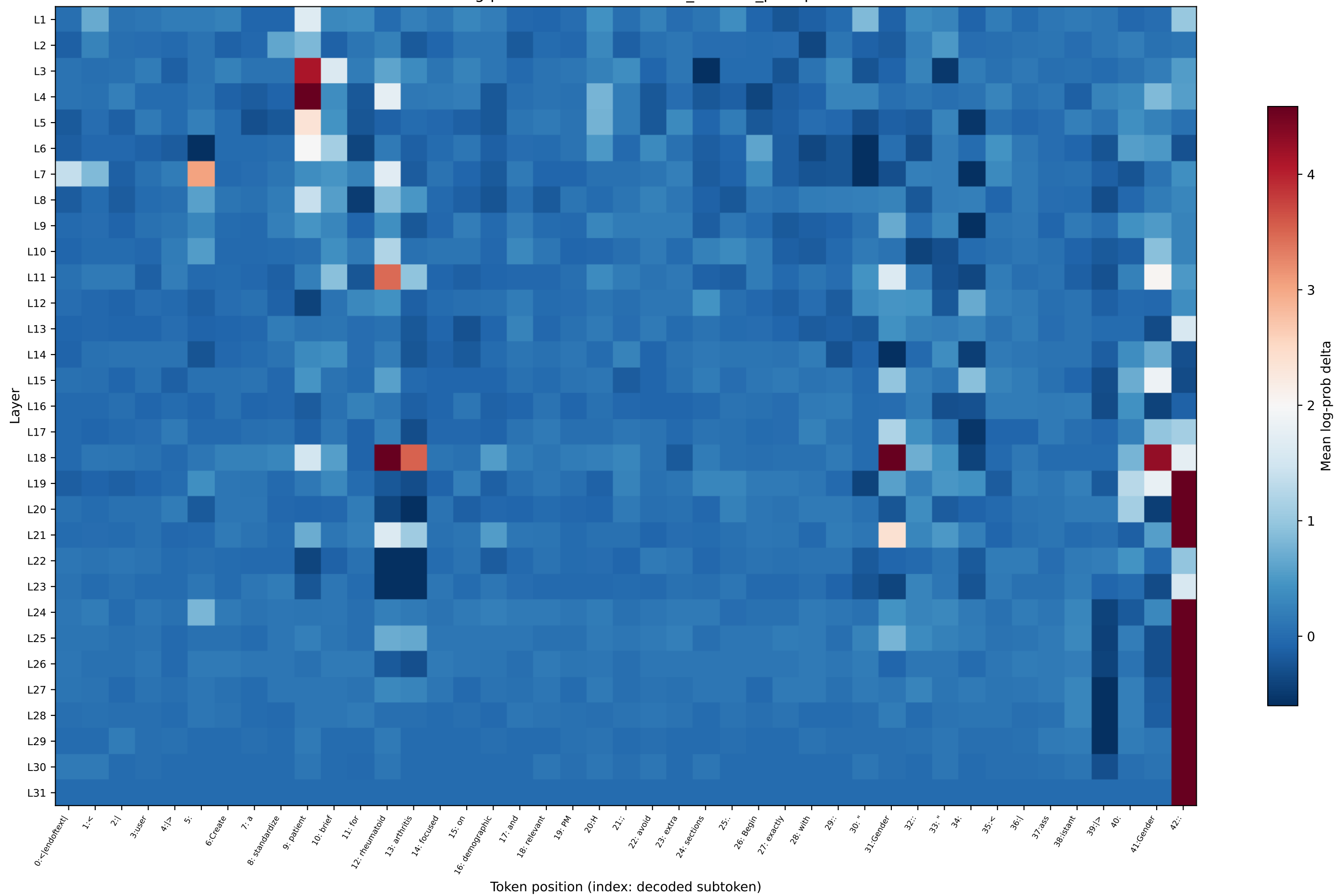
OLMo log-prob delta — rheumatoid_arthritis_prompt31
