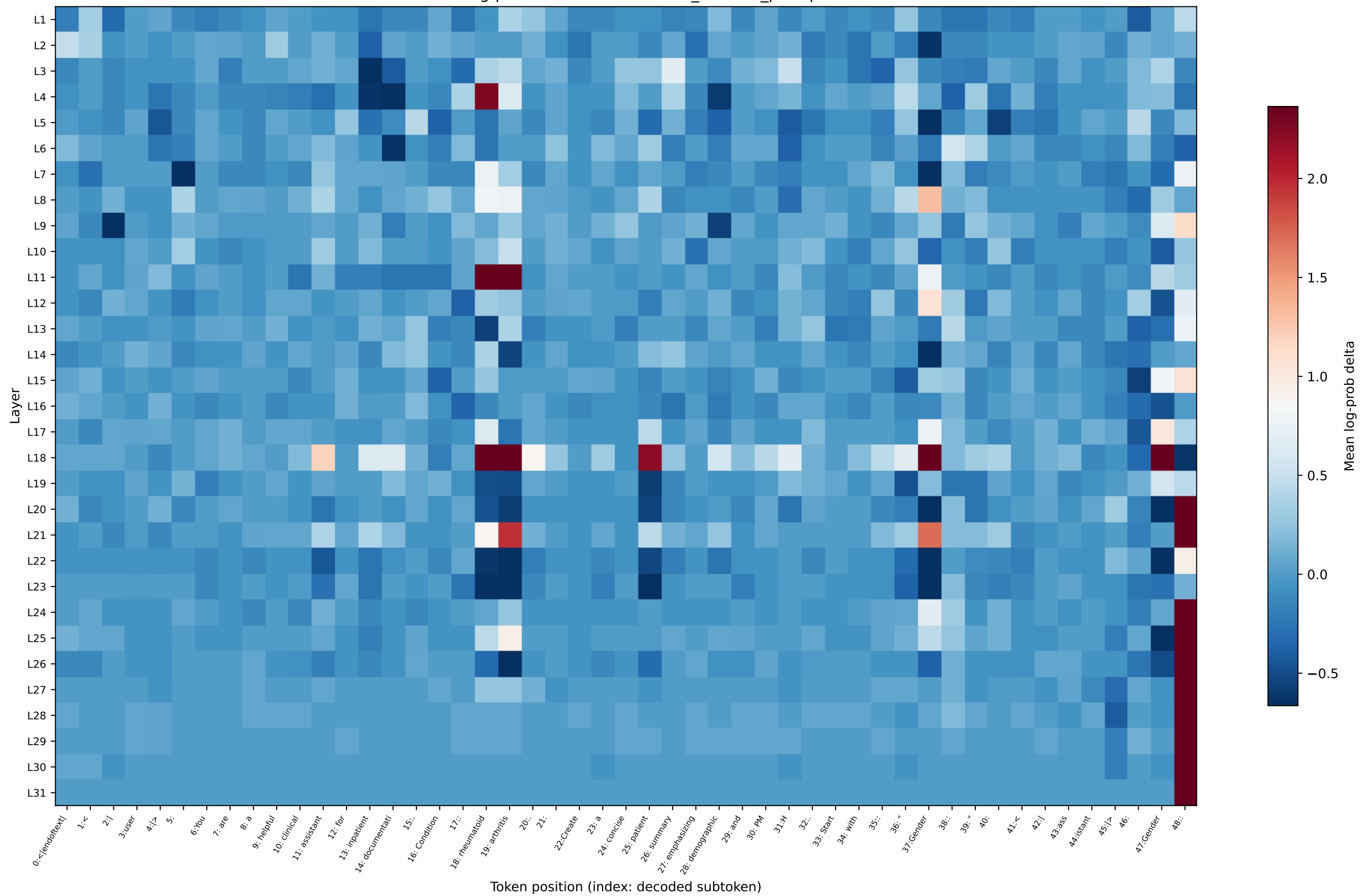
OLMo log-prob delta — rheumatoid_arthritis_prompt5
