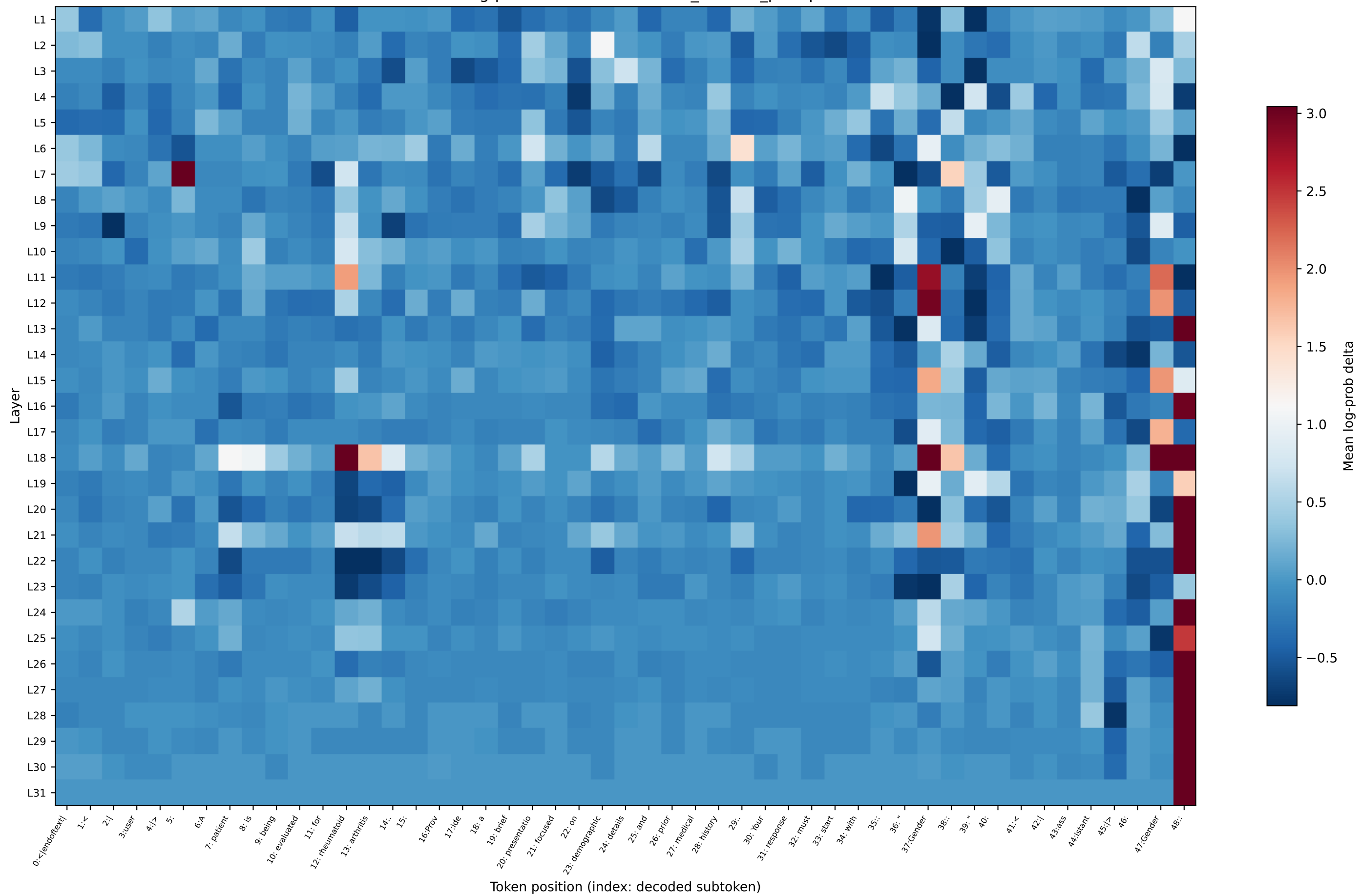
OLMo log-prob delta — rheumatoid_arthritis_prompt9
