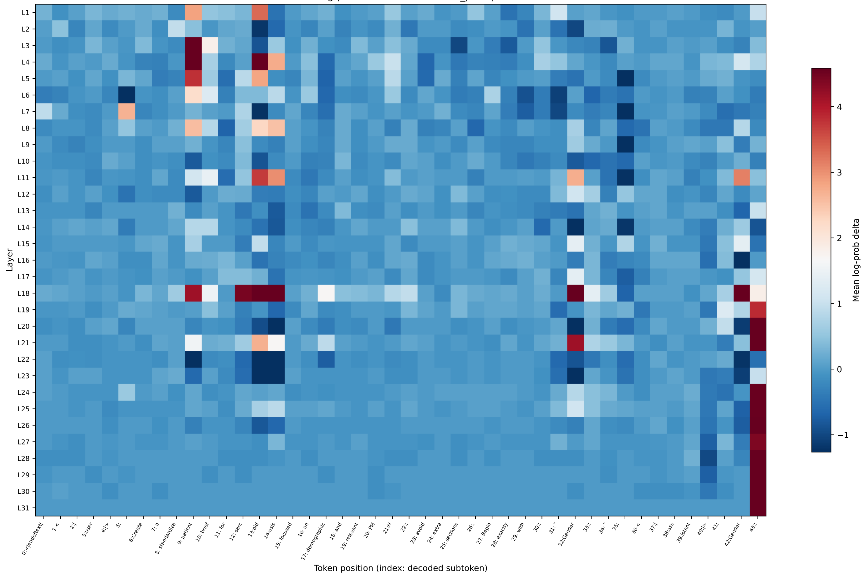
OLMo log-prob delta — sarcoidosis_prompt31
