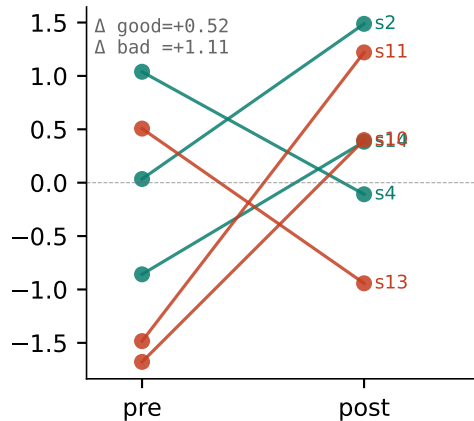
P1 CXCL13
