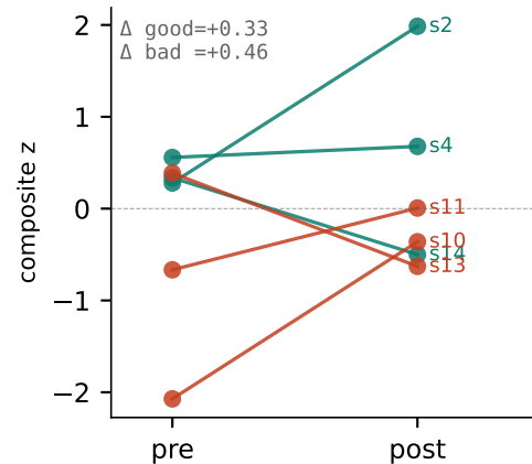
P3 Plasma-proxy
