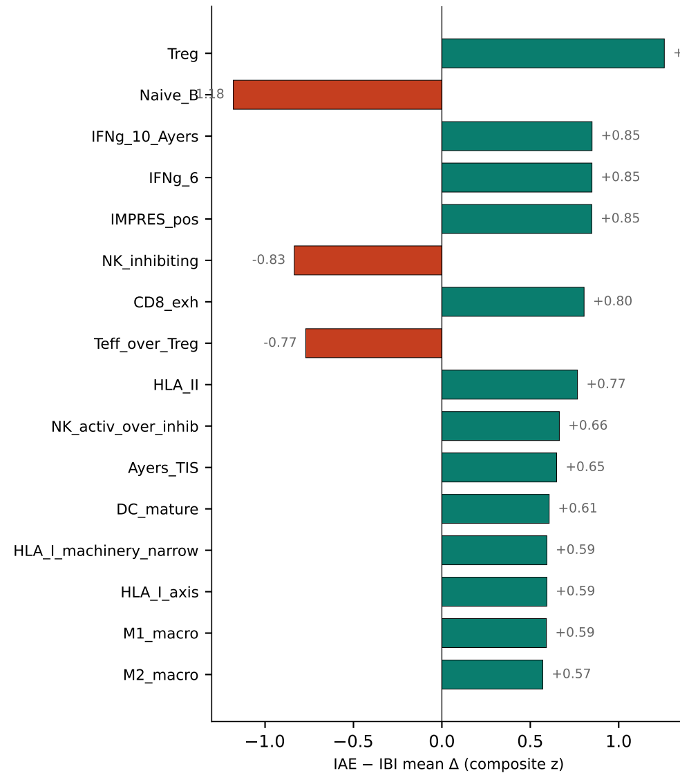
Composite level: IAE (n=2) vs IBI (n=3)
