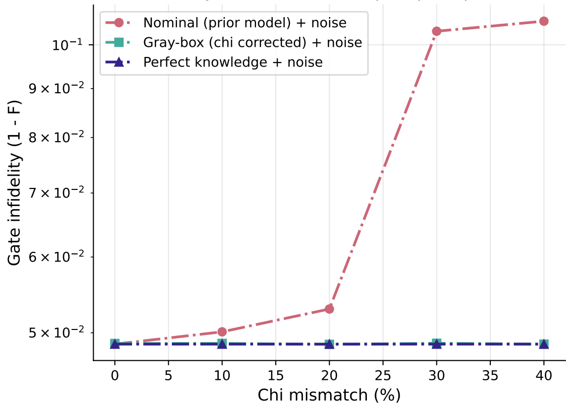
Noisy evaluation ( T_1=50 \mu\text{s} , T_\phi=40 \mu\text{s} )
