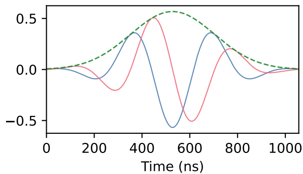
Multitone
