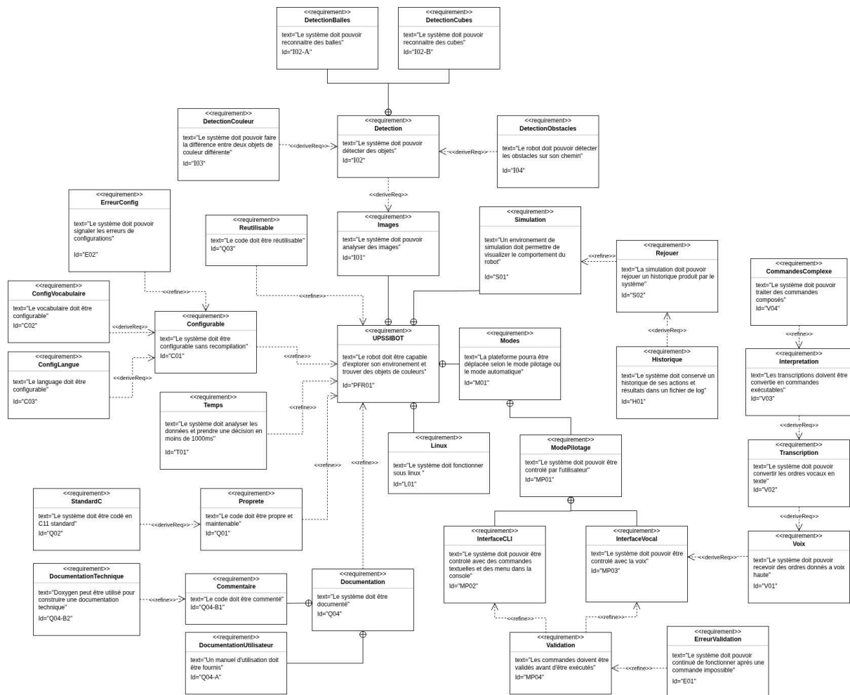
Figure 3: Diagramme des exigences de l'Upssibot
