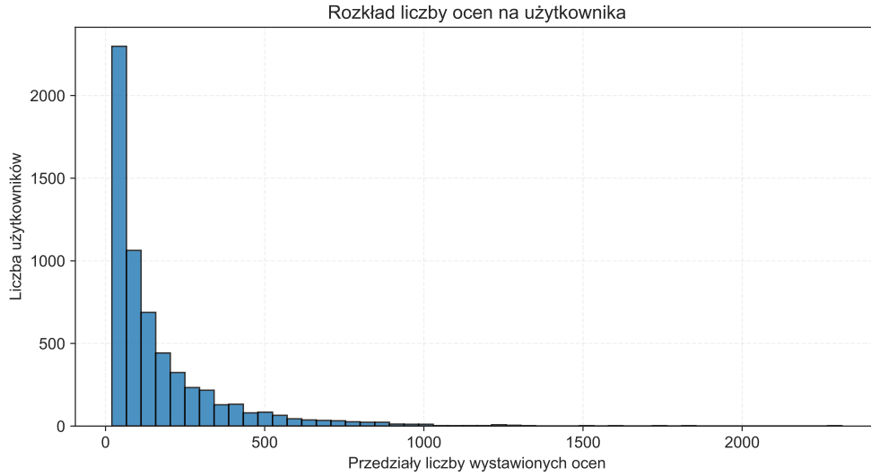
Rysunek 3: Rozkład liczby wystawionych ocen per użytkownik w zbiorze MovieLens 1M
