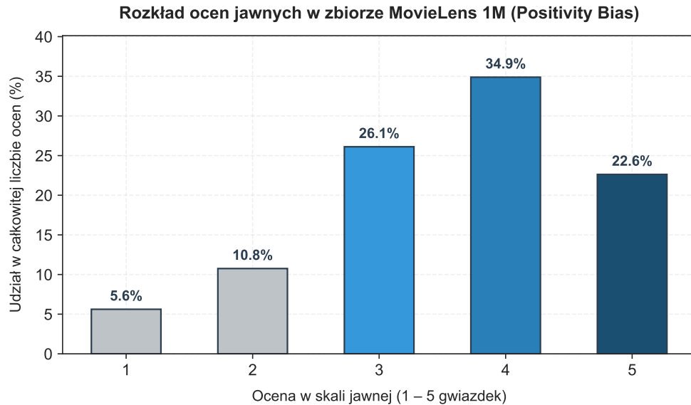
Rysunek 2: Rozkład ocen jawnych w zbiorze MovieLens 1M obrazujący efekt zjawiska positivity bias
