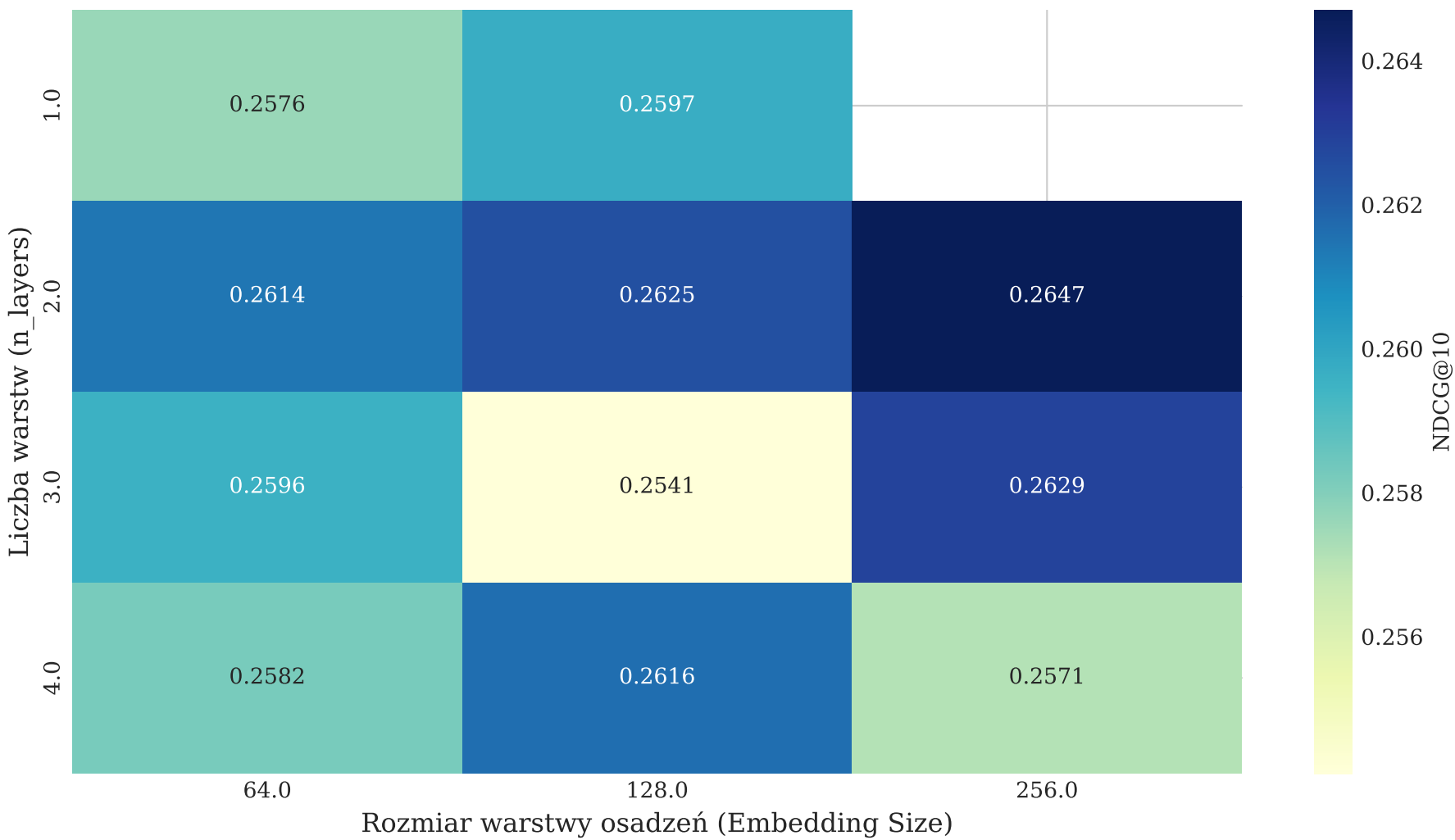
Wpływ liczby warstw (n_layers) i rozmiaru osadzeń na miarę NDCG@10 (LightGCN)
