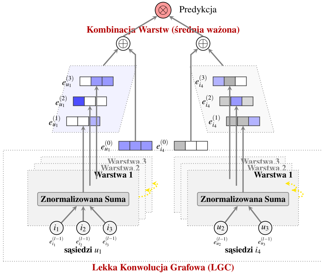
Rysunek 6: Architektura algorytmu LightGCN z uwzględnieniem propagacji warstwowej. Opracowanie własne na podstawie 91 .
